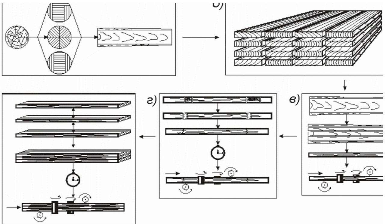
ис. 2. Структурна схема технологічного процесу виготовлення клеєного бруса а) розпилювання колоди на пиломатеріали; б) сушіння пиломатеріалів; в) зпилювання пиломатеріалів на ламелі потрібного розміру, калібрування ламелей зняття та видалення дефектів матеріалу, зрощування за довжиною, витримка калібрування ламелей; г) склеювання по пласті, витримка, калібрування бруса
