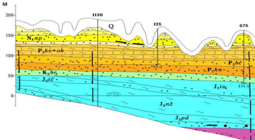
Рис. 2.6. Геологічний розріз
