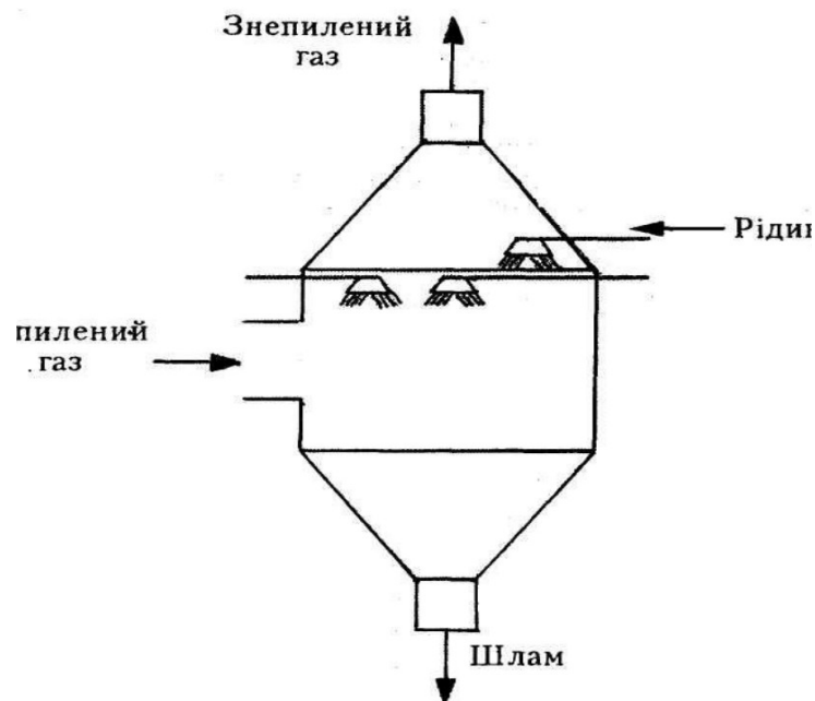
Рис. 5.1. Порожністий скрубер
