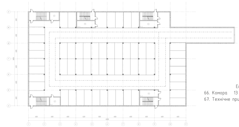
План паркінгу на відм. -3500 М
