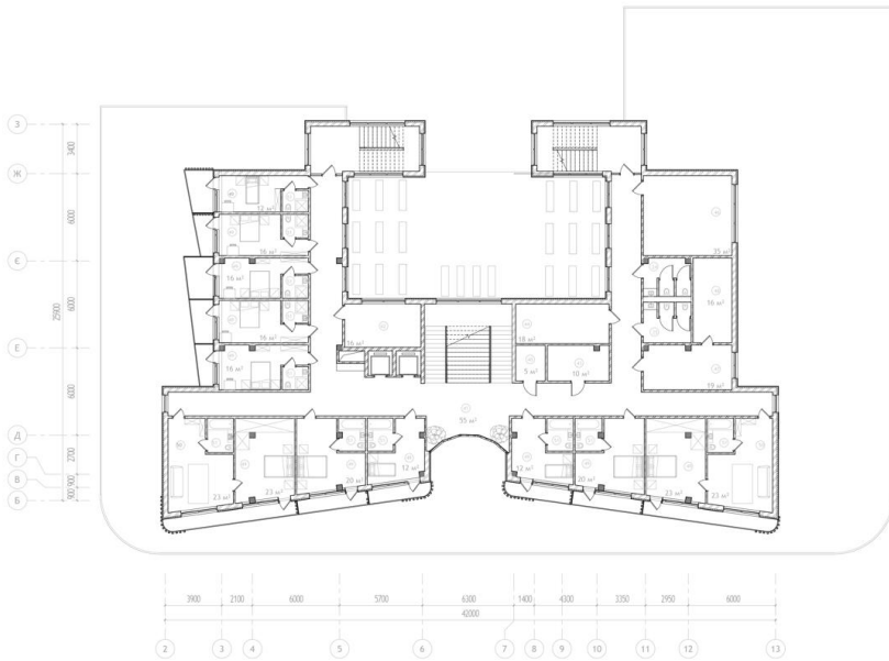
План на відм. +4.20 М 1:100
