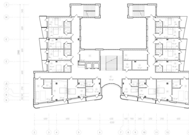
План на відм. +7.50 +10.80 +14.10 М 1:100
