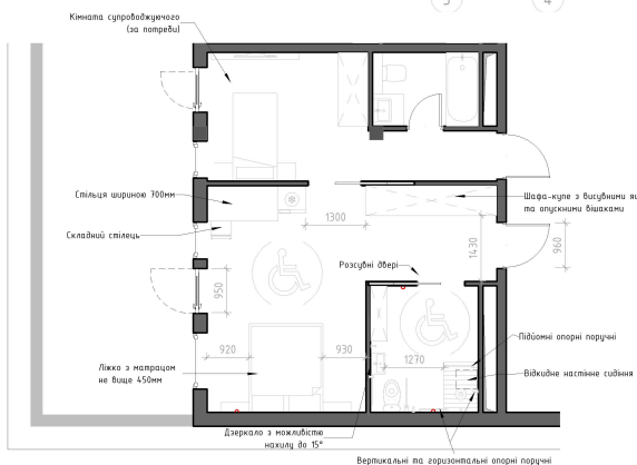
План на відм. +14.100
