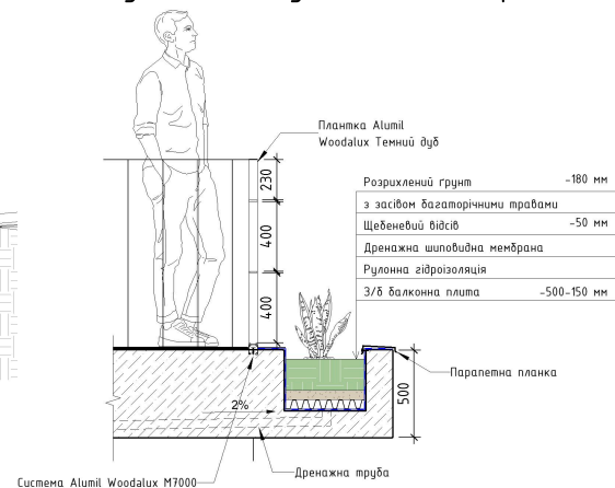
Вузол влаштування плантера
