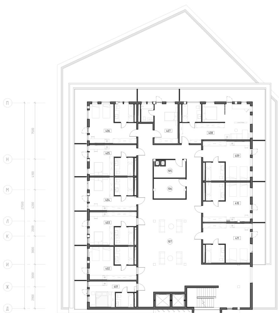
План на відм. +14.100
