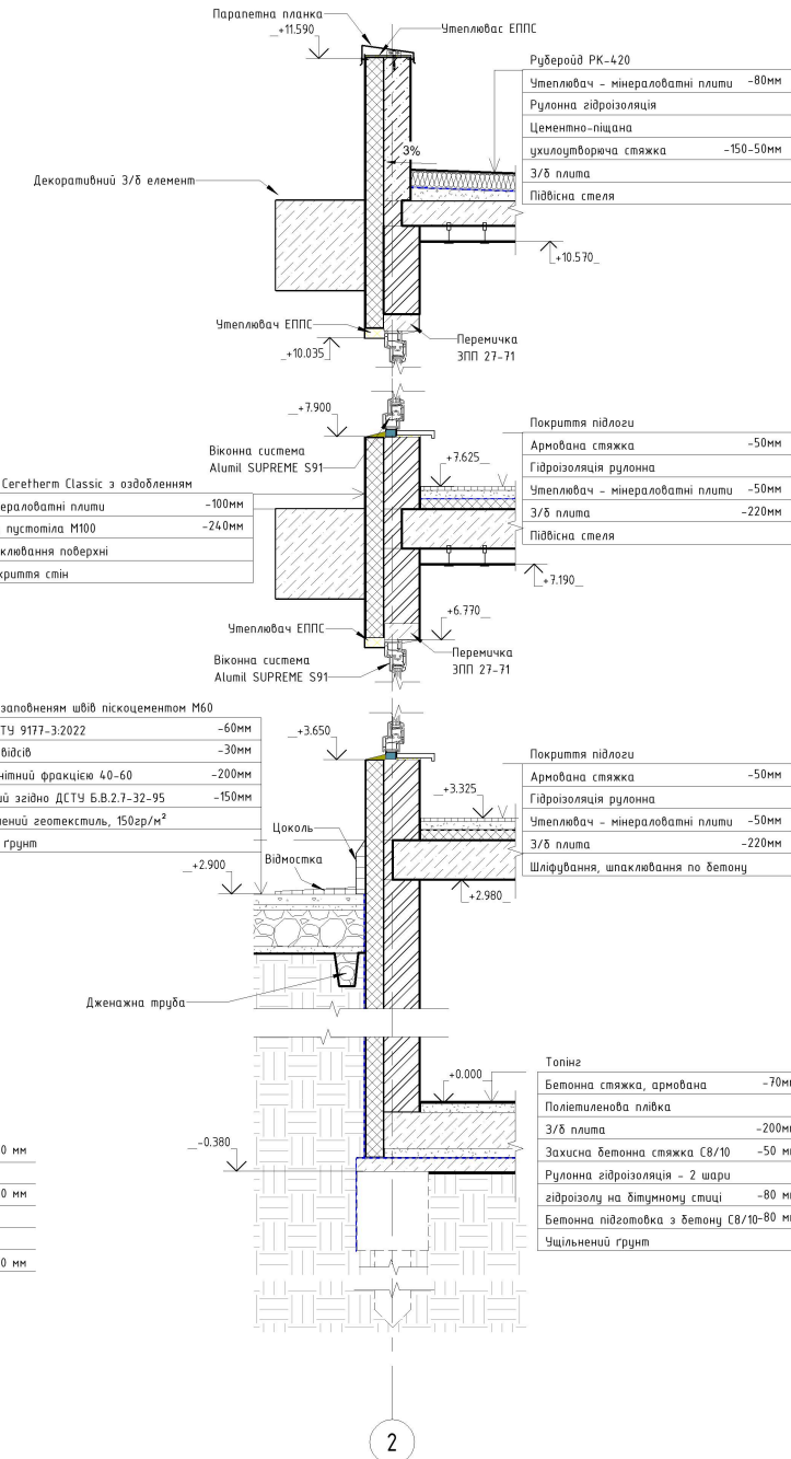
Розріз по стіні
