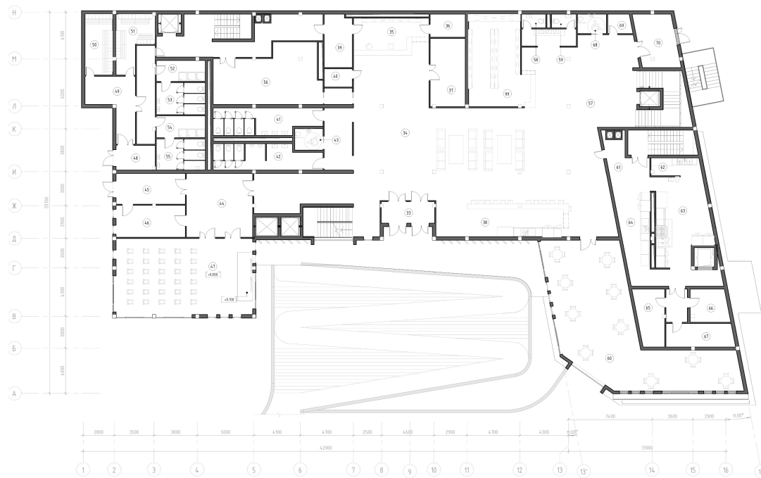
План на відм. +3.300
