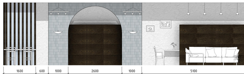
Розгортки інтер'єру
