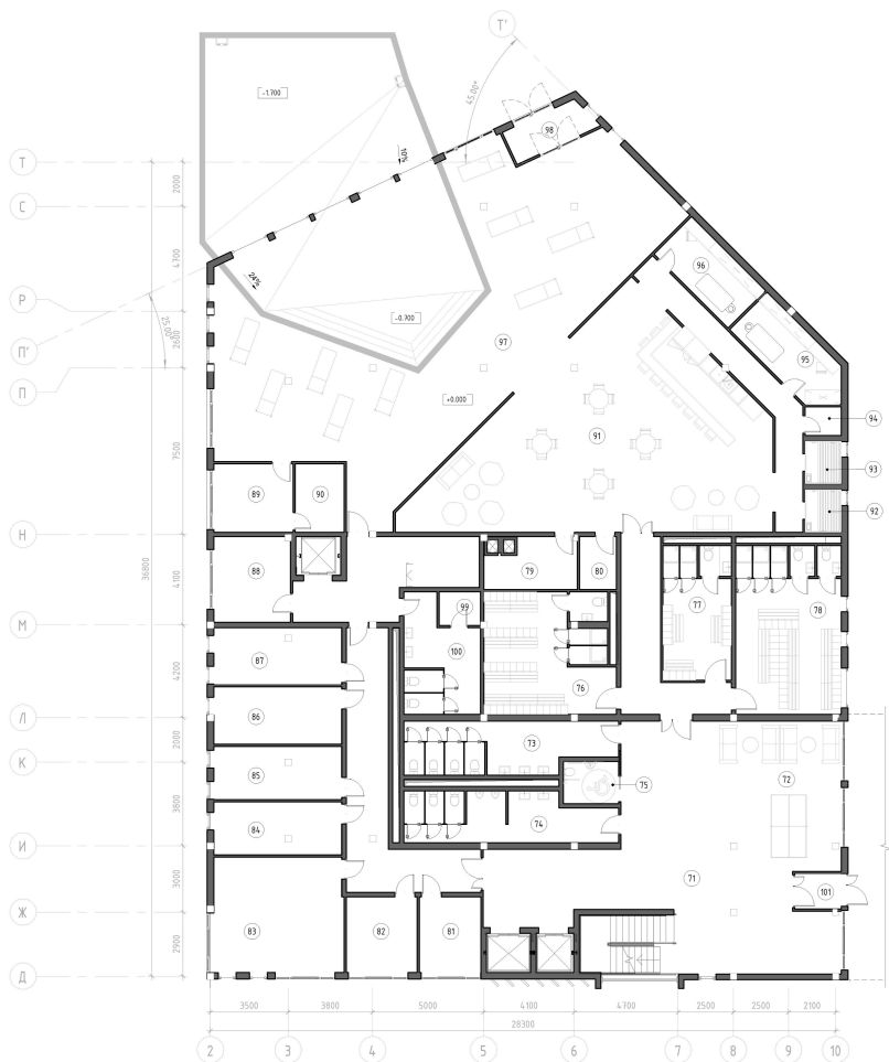
План на відм. +7.500
