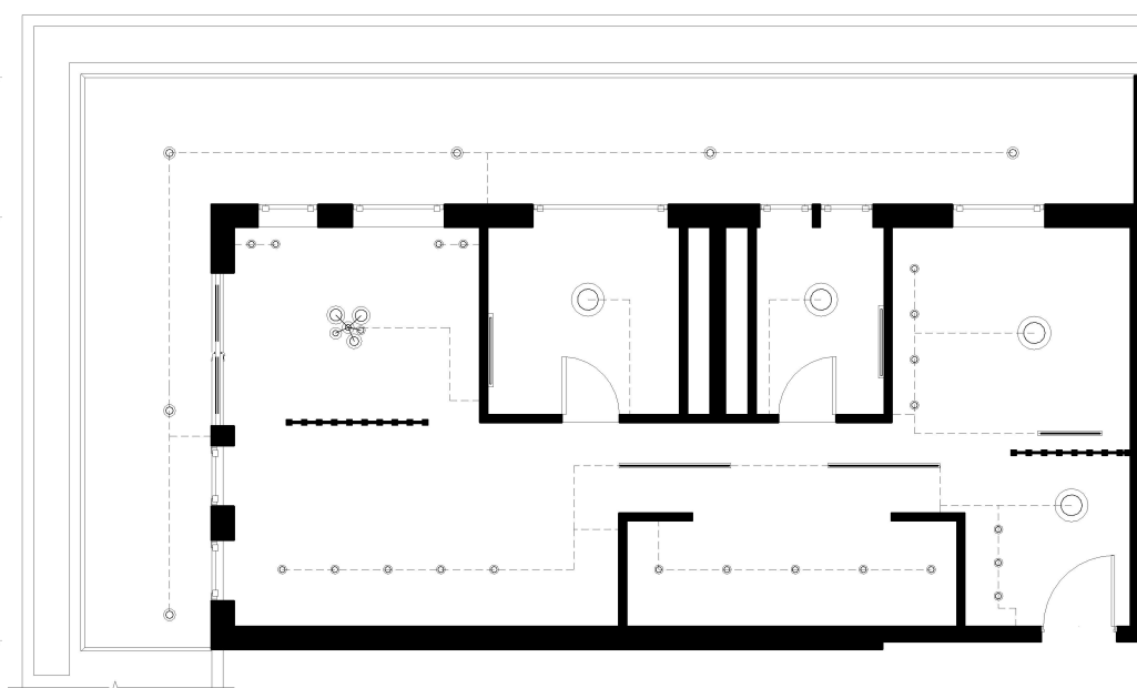
План освітлення апартаментів
