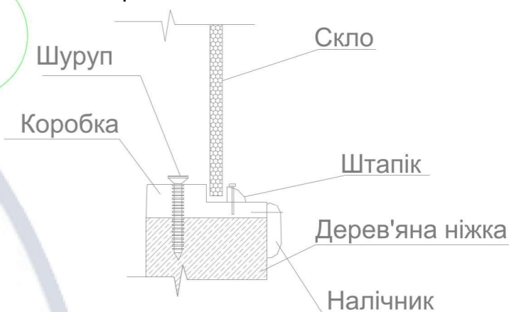
1. Кріплення скла, М1:5
