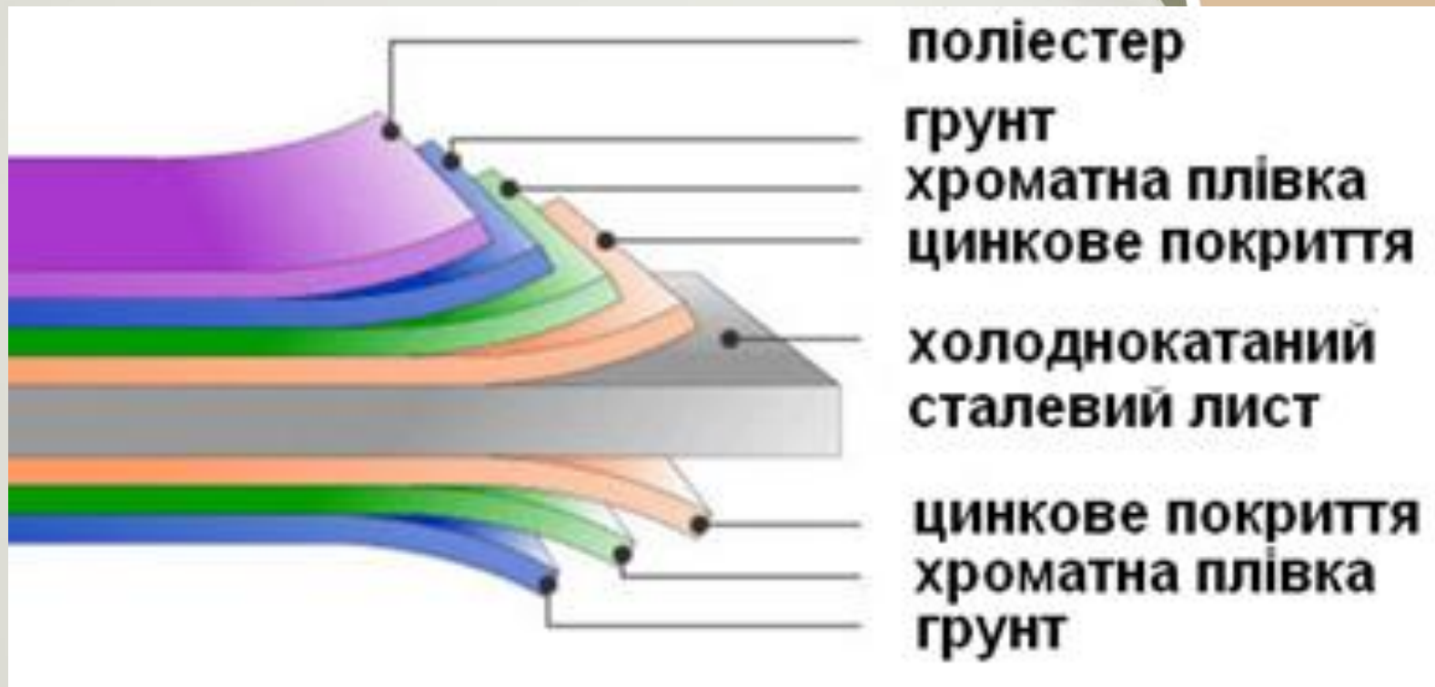
Рисунок 1 – Переріз листа профнастилу із захисним полімерним покриттям (поліестер)
