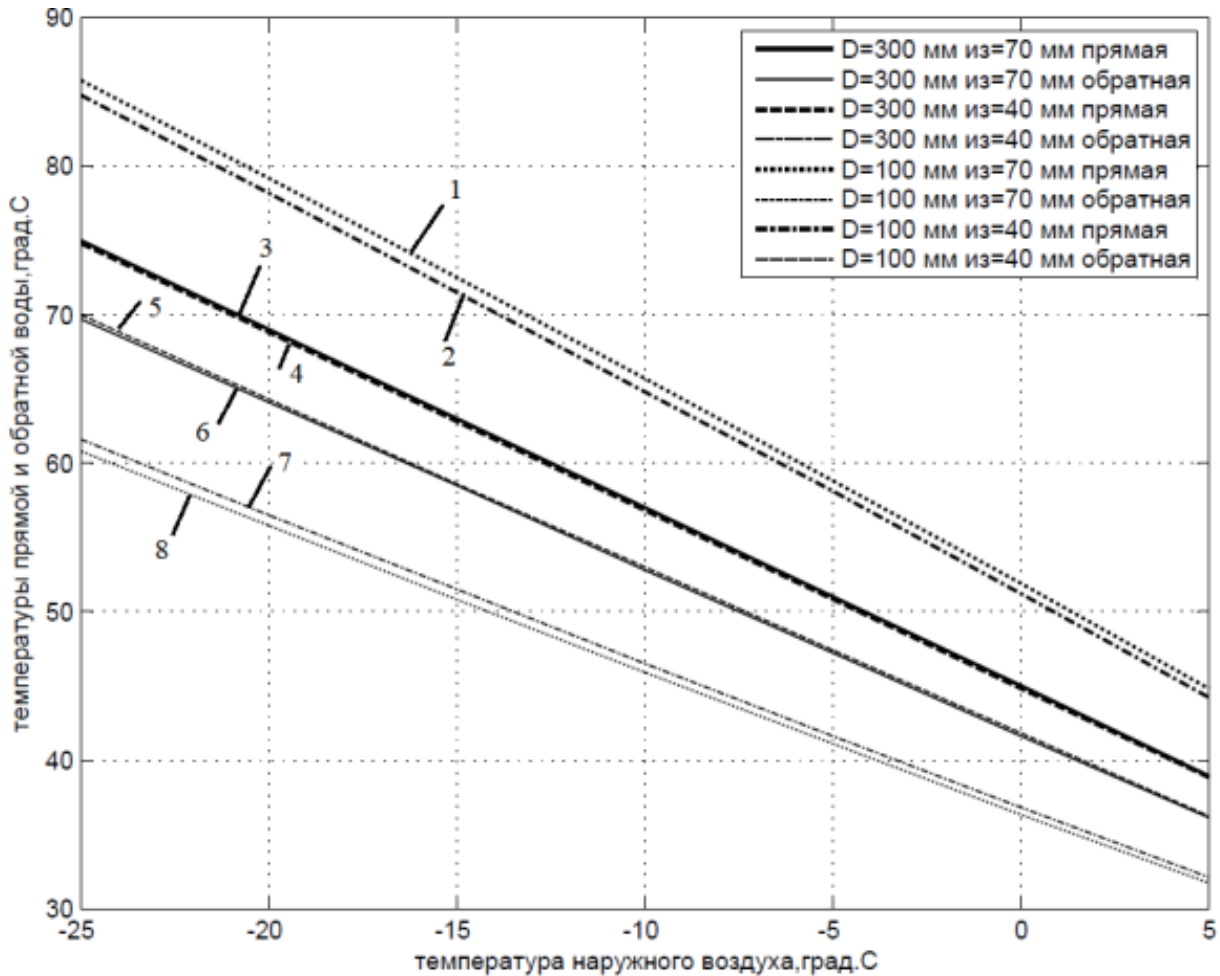
Рис. 2. Залежність температури теплоносія від температури зовнішнього повітря ( Q_{max} = 600 кВт; K \cdot F = 12 кВт/К): 1 – d=100 мм, \delta=70 мм (пряма вода); 2 – d=100 мм, \delta=40 мм (пряма вода); 3 – d=300 мм, \delta=70 мм (пряма вода); 4 – d=300 мм, \delta=40 мм (пряма вода); 5 – d=300 мм, \delta=40 мм (обратна вода); 6 – d=300 мм, \delta=70 мм (обратна вода); 7 – d=100 мм, \delta=40 мм (обратна вода); 8 – d=100 мм, \delta=70 мм (обратна вода)
