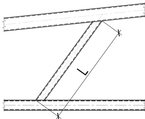
Рисунок Д.3.7. — Визначення довжини елементів замкнутого перерізу
