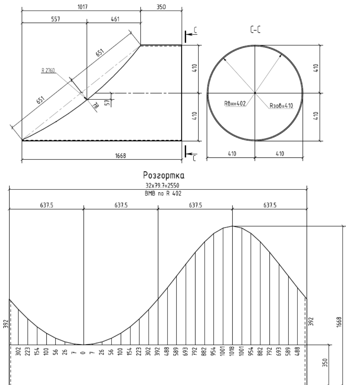
Рис. 5. Зображення вальцьованих деталей
