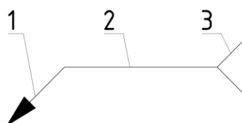
Рисунок Д.4.1 — Умовне позначення зварного з'єднання за ДСТУ ISO 2553:2019. Де: 1 — стрілка, що застосовується для вказання з'єднання (вказує на лінію примикання деталей, що зварюються); 2 — опорна лінія, на якій вказують основні знаки (тип і розміри зварного шва та підготовка деталей для з'єднання); 3 — «хвіст» опорної лінії для наведення додаткової інформації.
