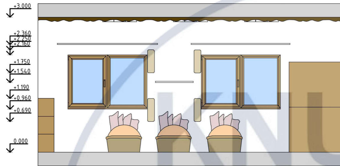
Розгортка 1-2
