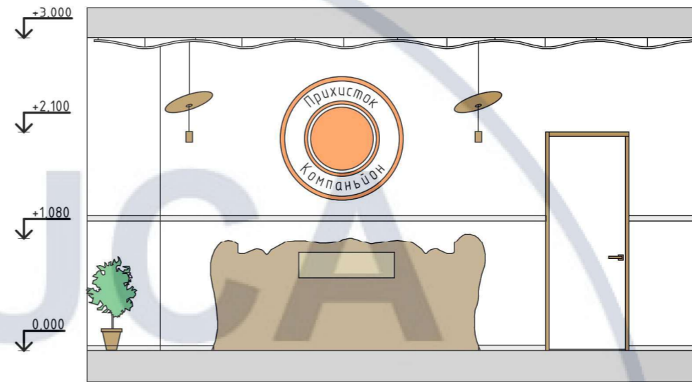
Розгортка 2-3
