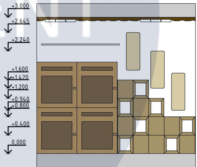
Розгортка 4-1
