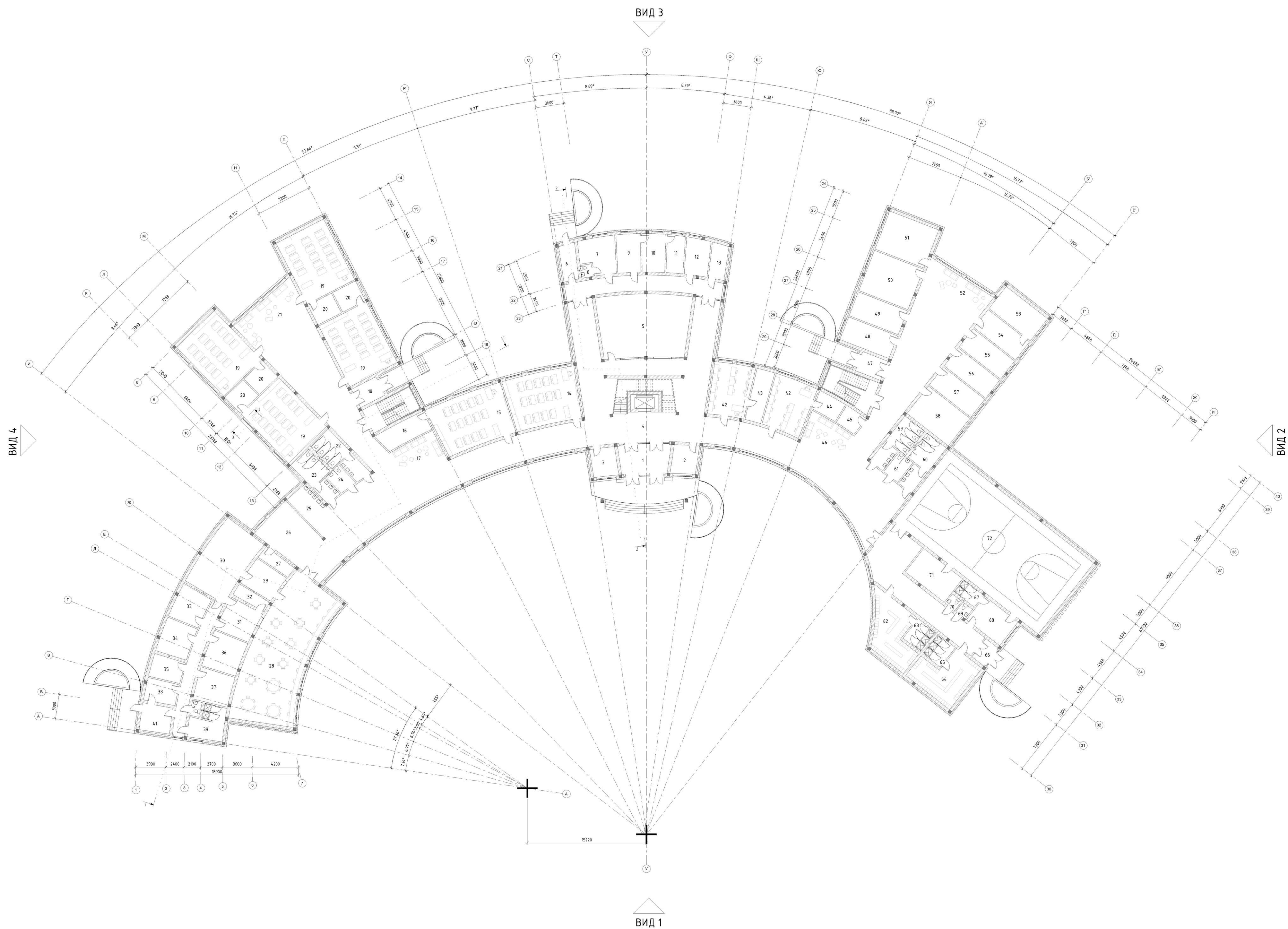
ПЛАН НА ВІДМІТЦІ +0,000 М 1:200
