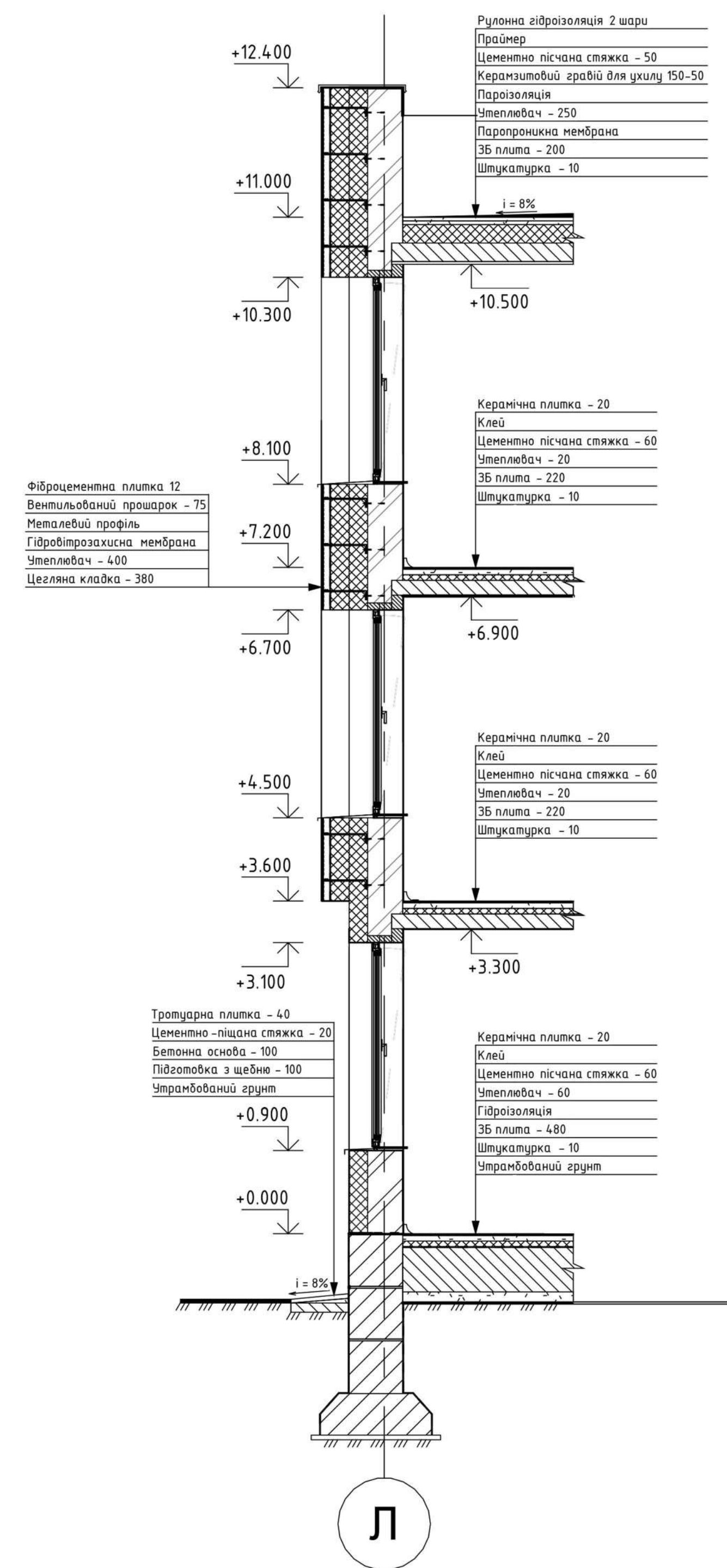
P03PI3 3 - 3 M 1:20
