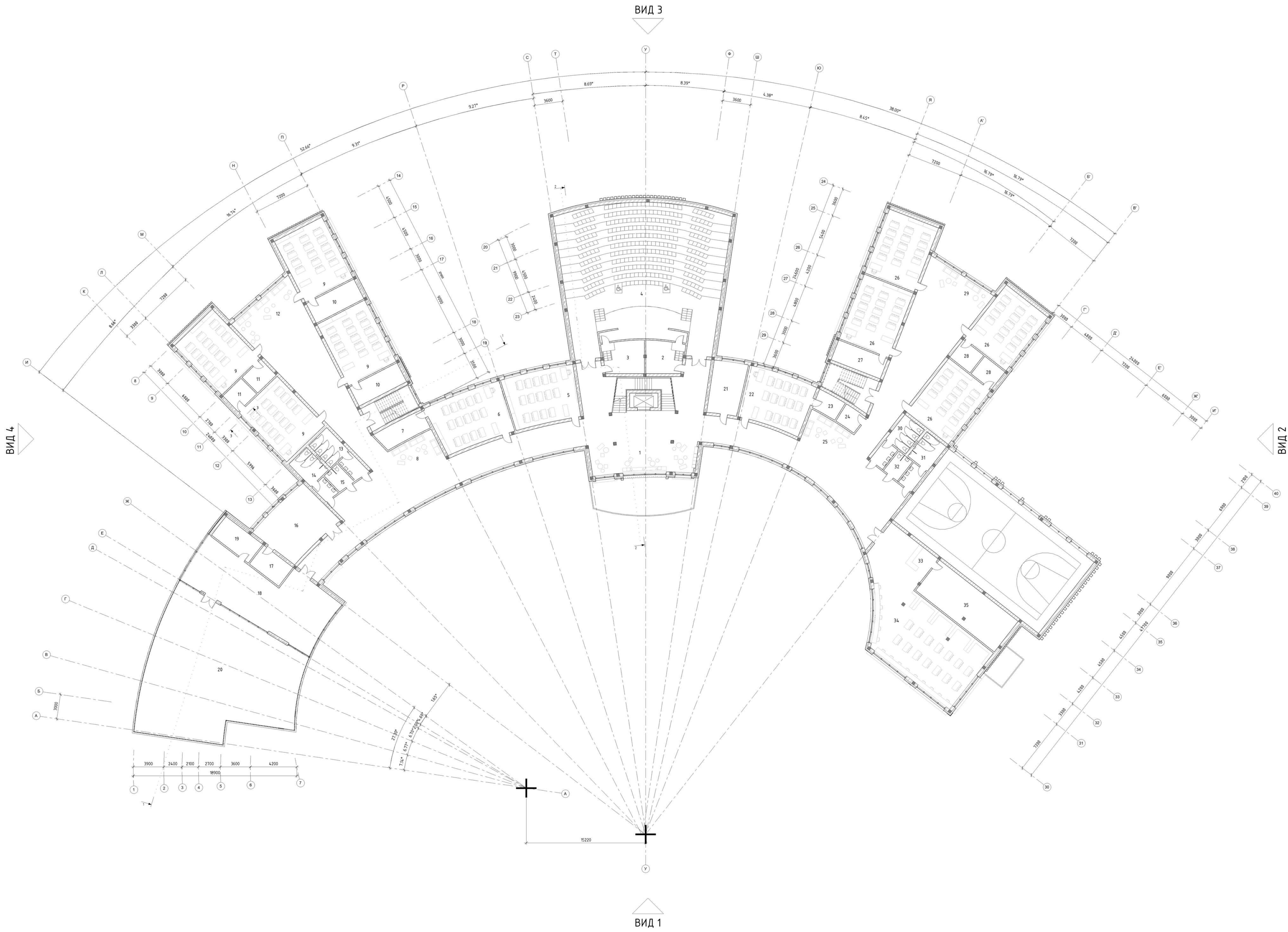
ПЛАН НА ВІДМІТЦІ +3,600 М 1:200
