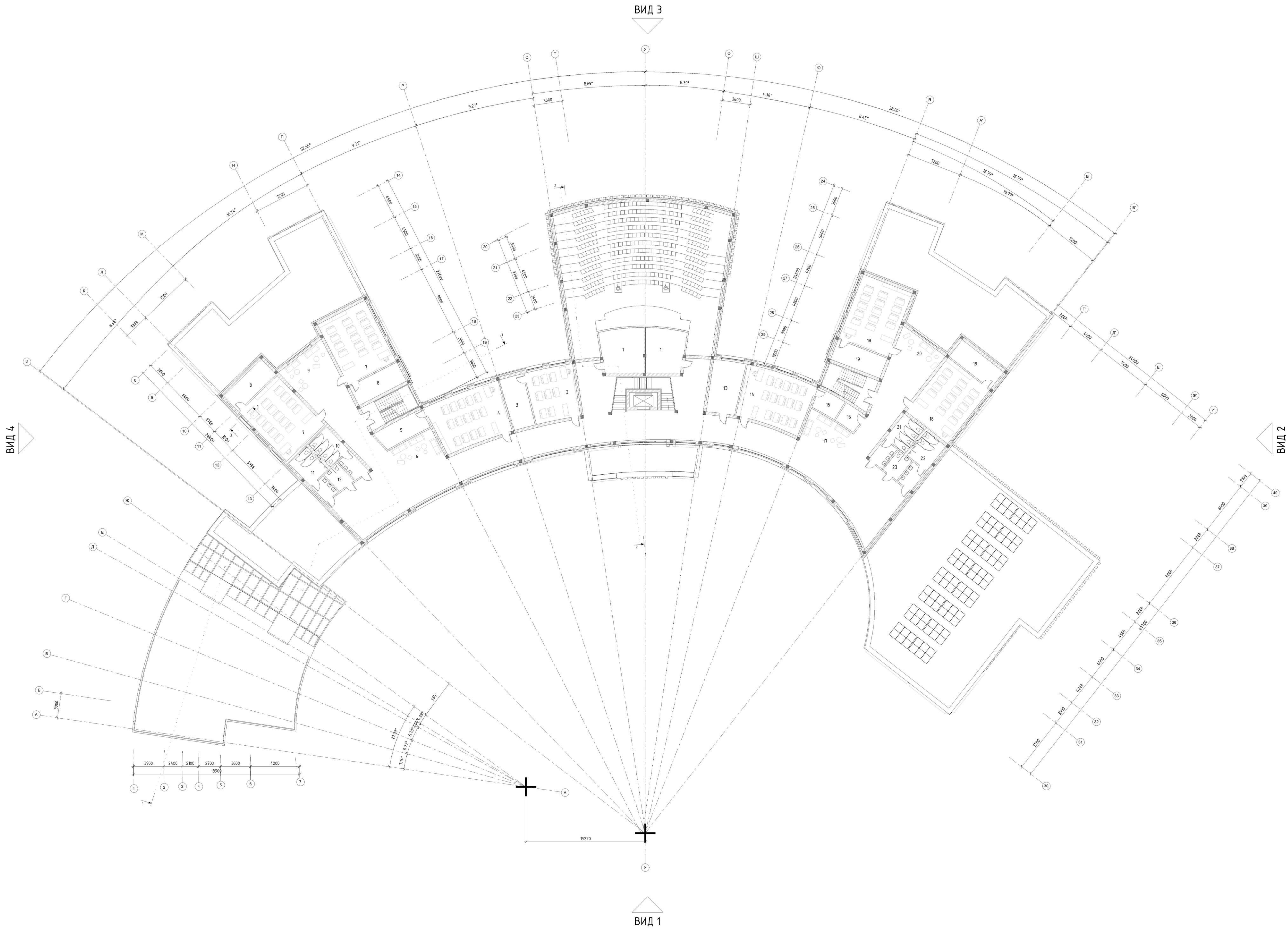
ПЛАН НА ВІДМІТЦІ +7,200 М 1:200
