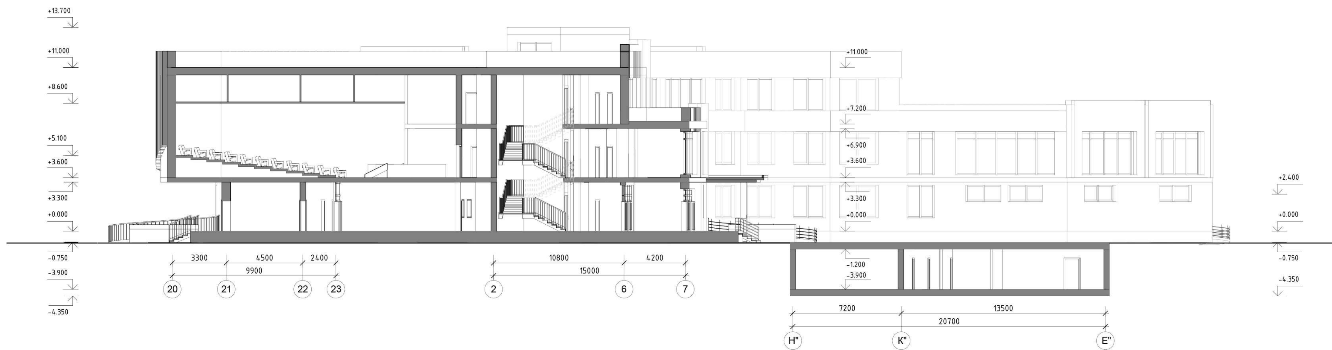
P03PI3 2-2 M 1:200
