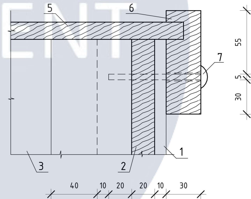
Вузол 3. Механізм відкриття
