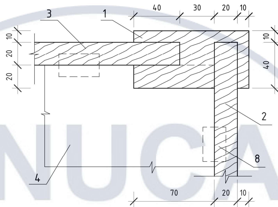
Вузол 1. З'єднання дна, стінок та ніжки
