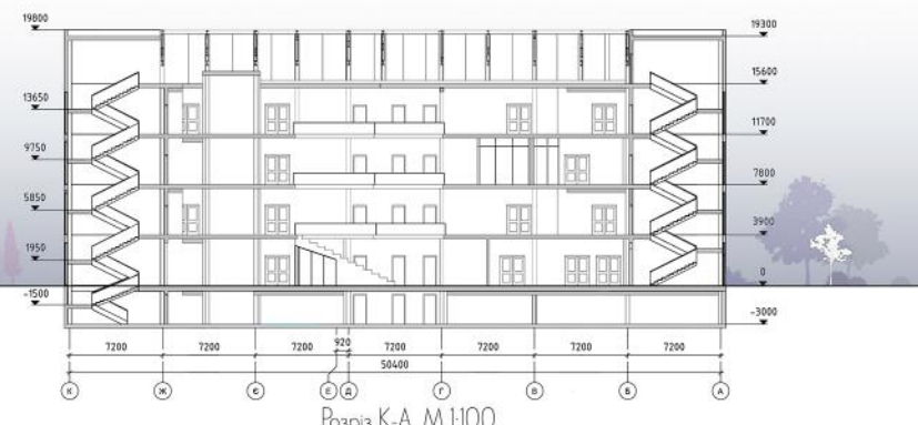
Розріз К-А М 1:100
