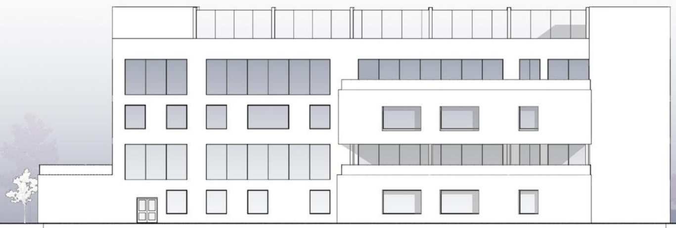
Фасад Л-А
