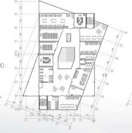
План поверху на відмітці +3.900 М 1:200
