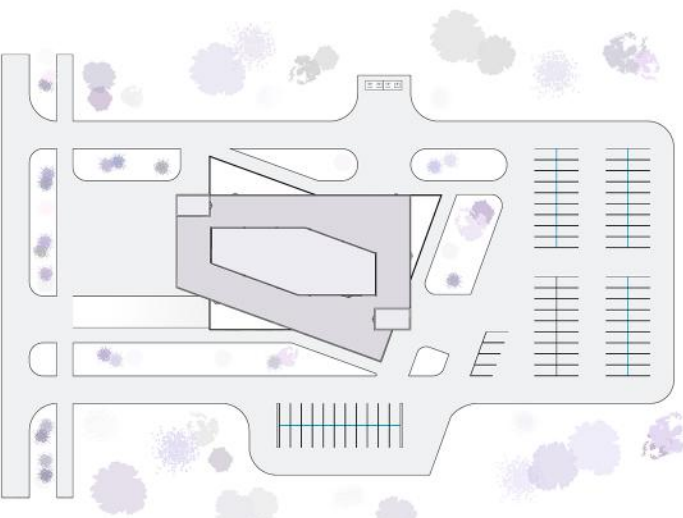
Генеральний план 1:500
