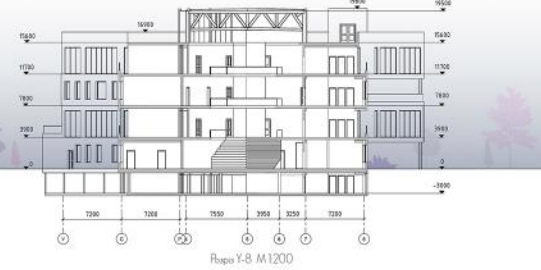
Розріз Y-B М 1:200
