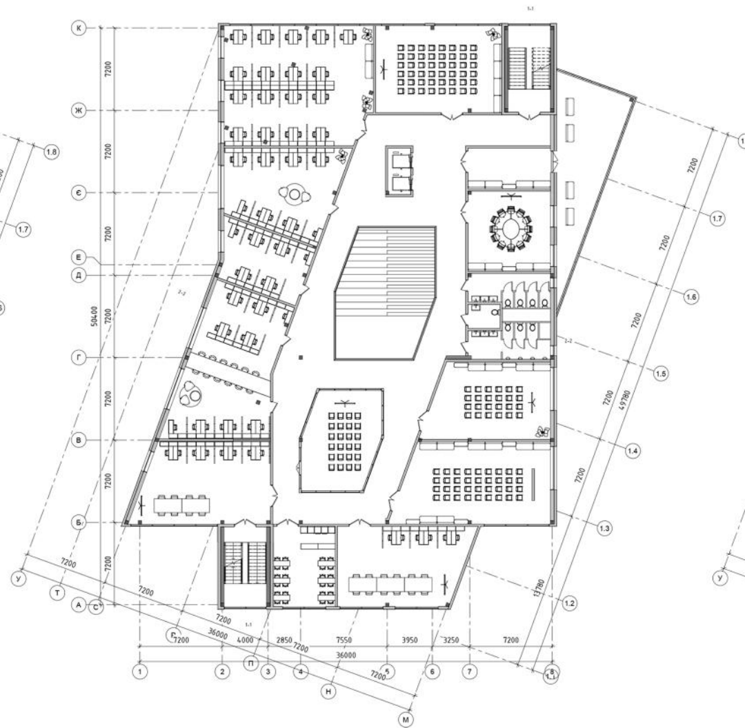
План поверху на відмітці +7.800
