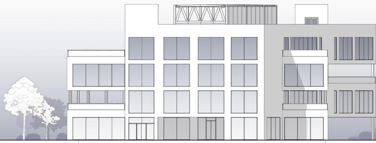
Фасад 1-7
