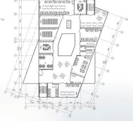
План поверху на відмітці +11.700 М 1:200
