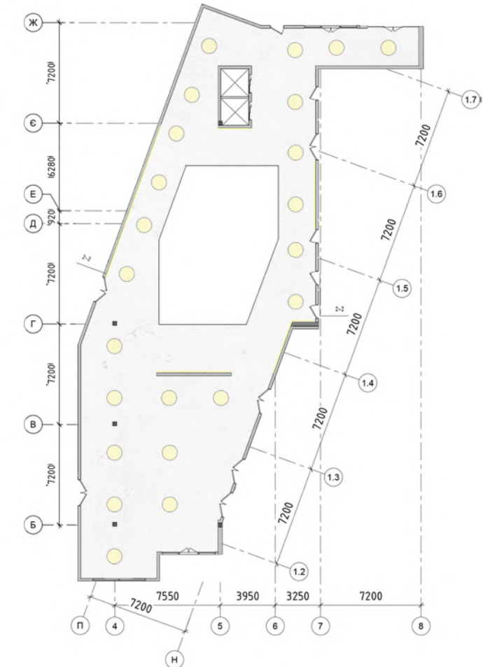
План освітлення М 1:50
