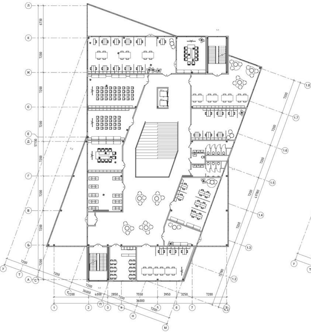
План поверху на відмітці +3.900
