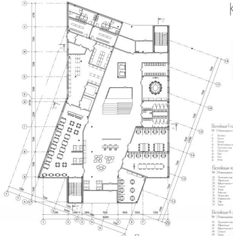
План поверху на відмітці 0.000 М 1:100
