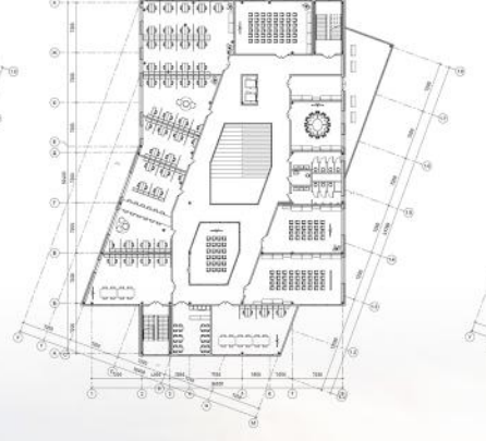
План поверху на відмітці +7.800 М 1:200
