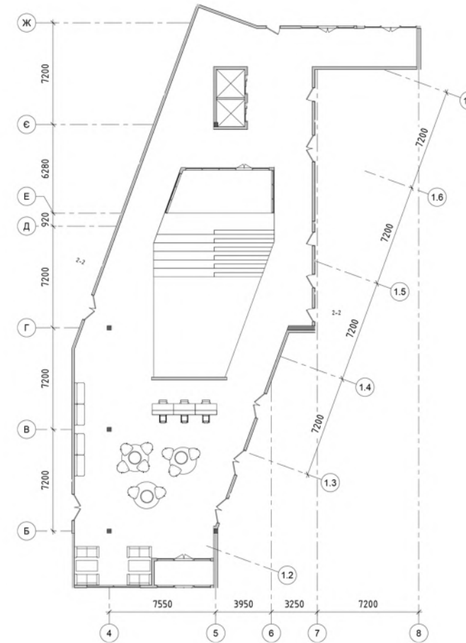
План атриумного простору М 1:50
