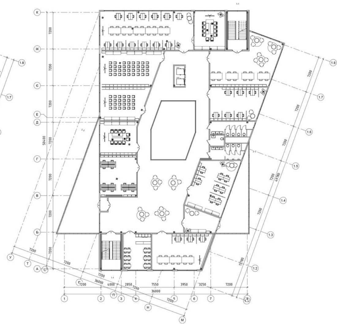
План поверху на відмітці +11.700
