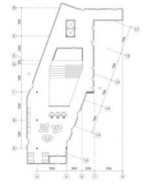
План спільного простору М 1:50
