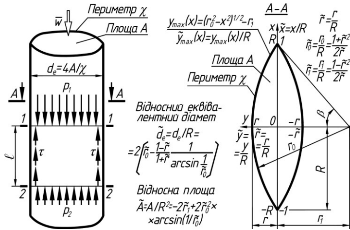
Рис 1. Двокутний канал
