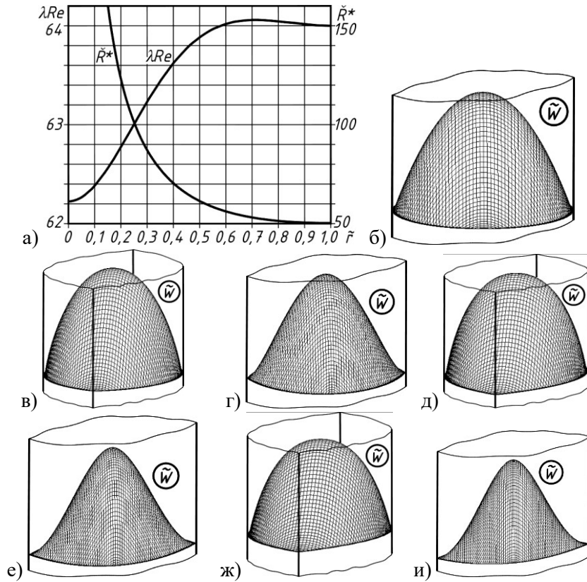
Рис. 2. Профілі швидкості:
