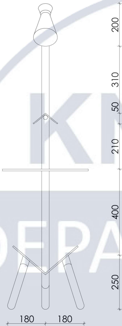
Вид спереду
