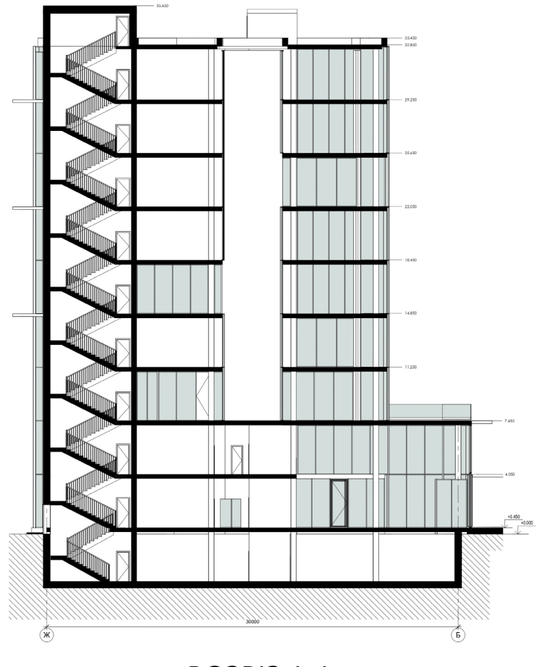
PO3PI3 1-1
