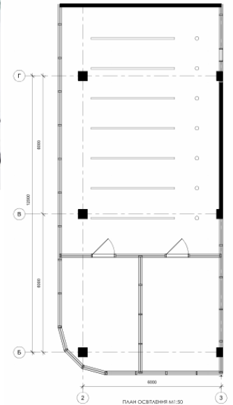
План освітлення
