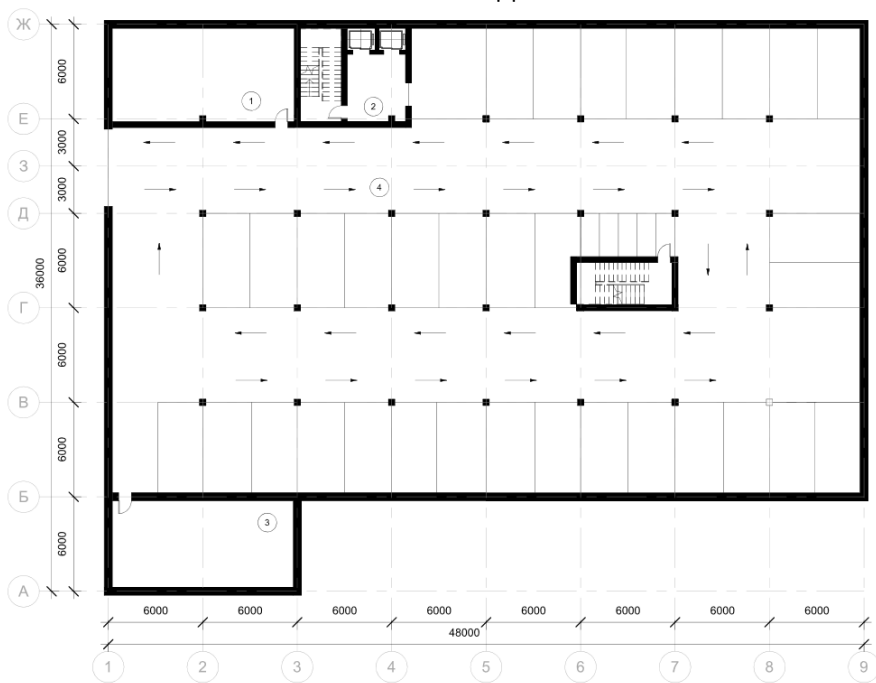
ПЛАН 0 ПОВЕРХУ
