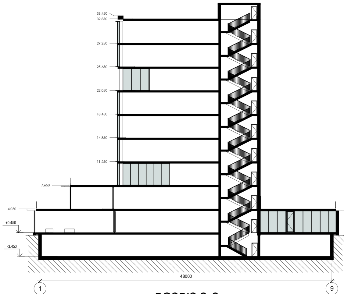
PO3PI3 2-2
