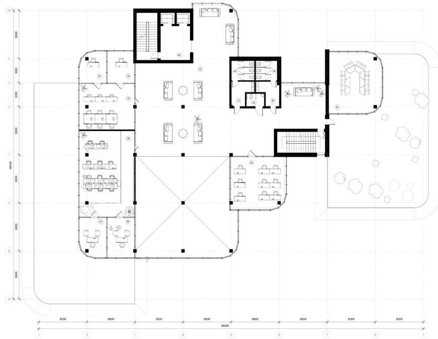
ПЛАН 2 ПОВЕРХУ
