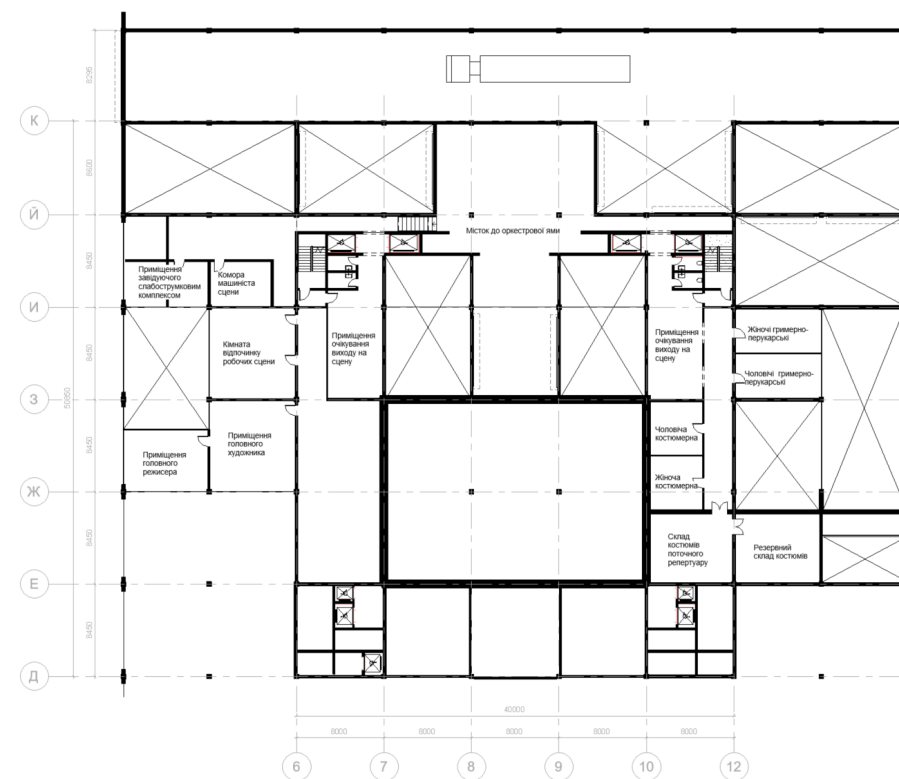
План в рівні +/-3.30
