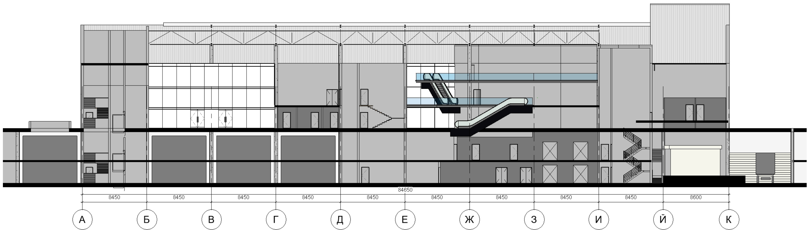
Розріз 2-2
