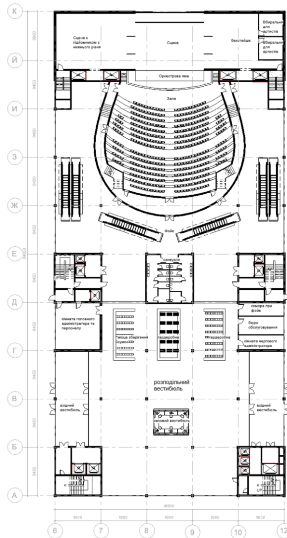
План в рівні +/-0.00
