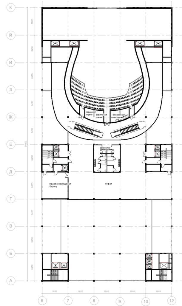
План в рівні +13.40
