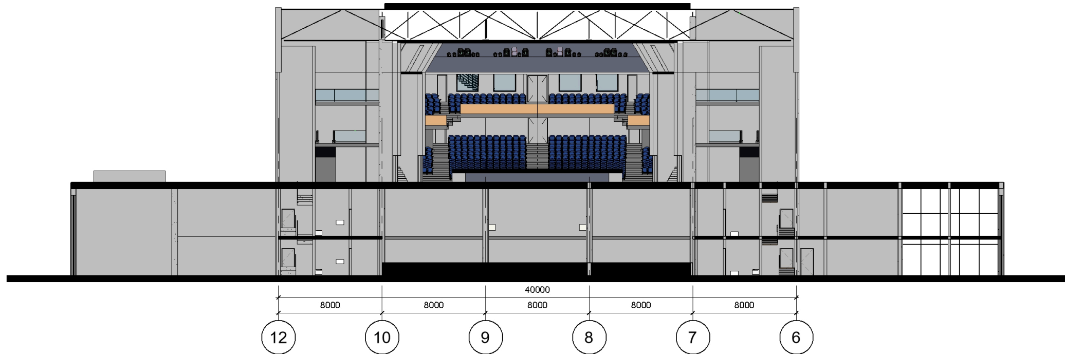
Розріз 1-1
