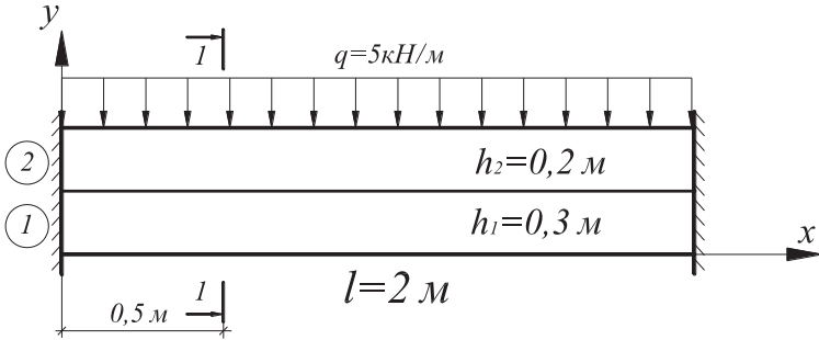
Рис. 11. Двошарова пластина, жорстко защемлена по бічних гранях
