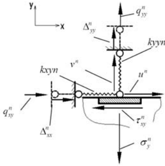
Рис. 7. Граничні умови на n - й прямій
