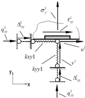
Рис. 8. Граничні умови на 1 - й прямій:
