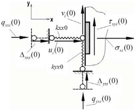
Рис. 5. Граничні умови на лівій грані пластини
