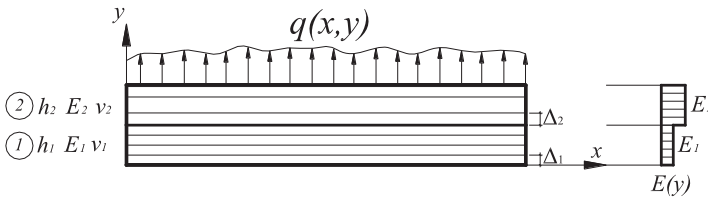
Рис. 3. Розрахункова модель
