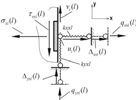
Рис. 6. Граничні умови на правій грані пластини
