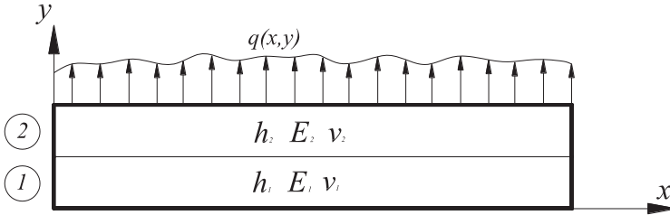
Рис. 2. Плоска деформація пластини.
