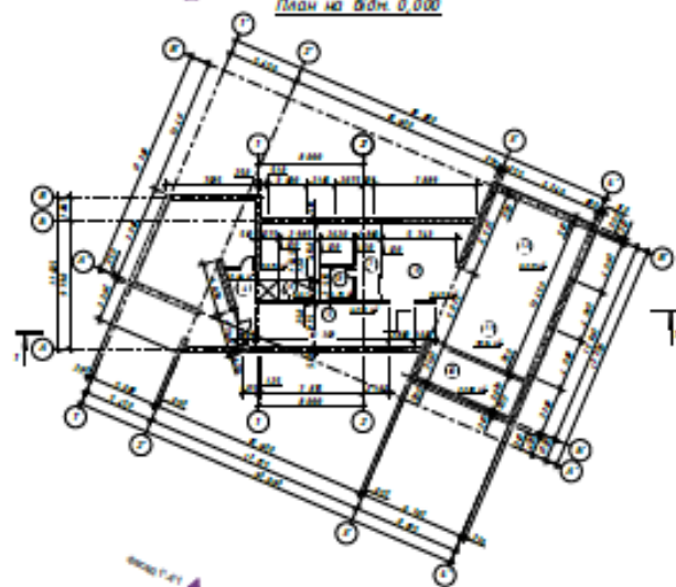
План на вѣн 0.000
