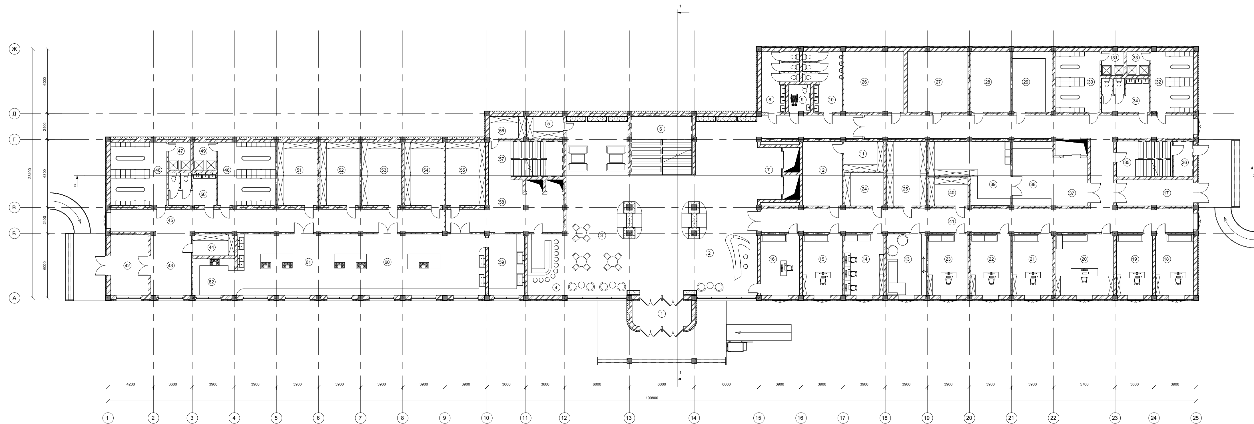
План на відмітці +0.000 М 1:200
