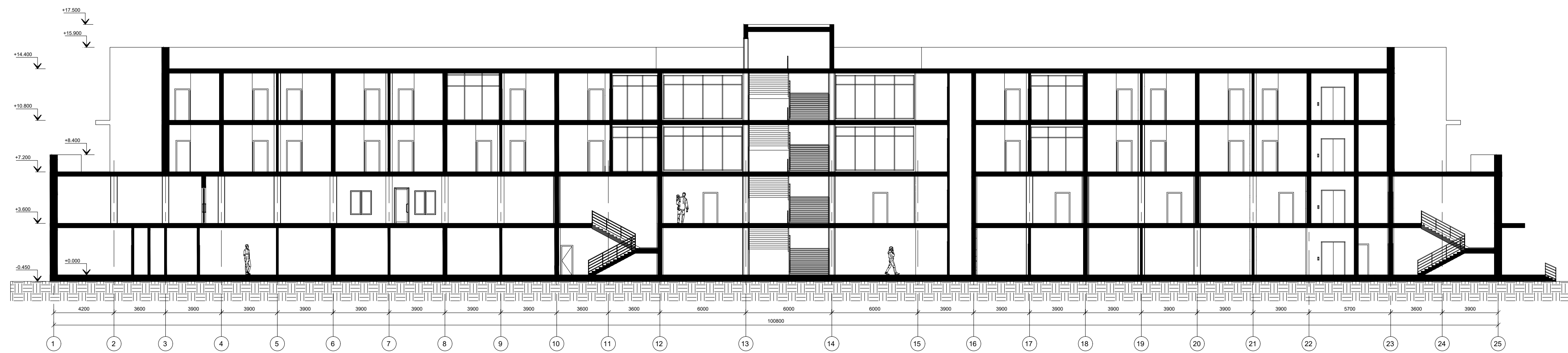
Розріз 2-2 М 1:200
