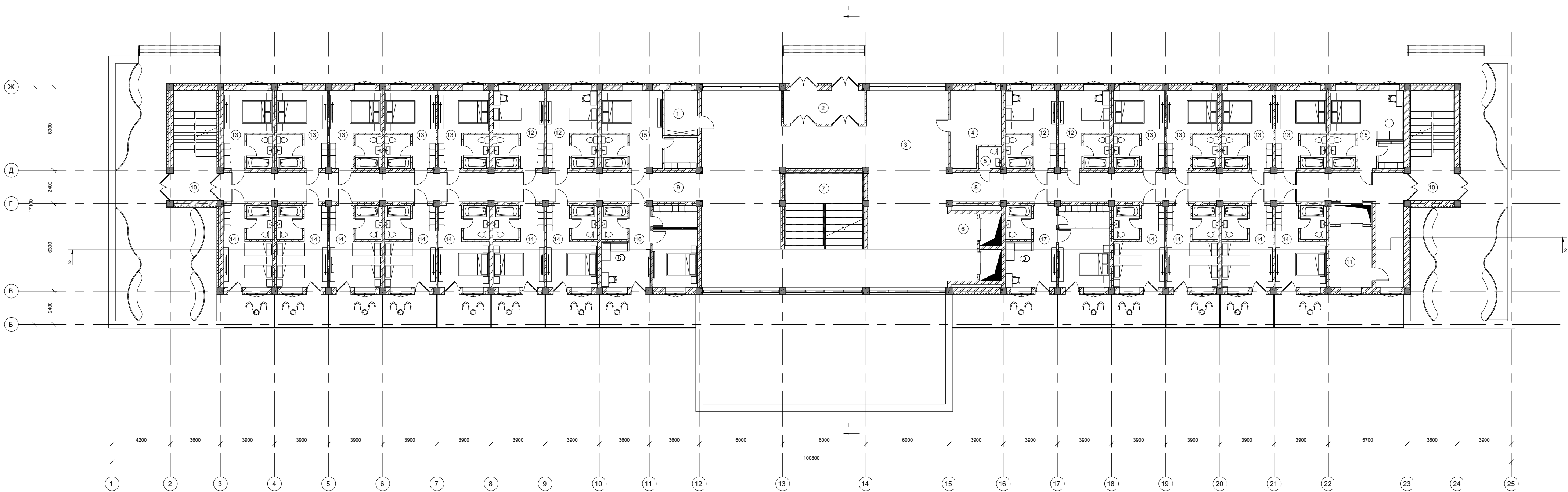
План на відмітці +7.200 М 1:200
