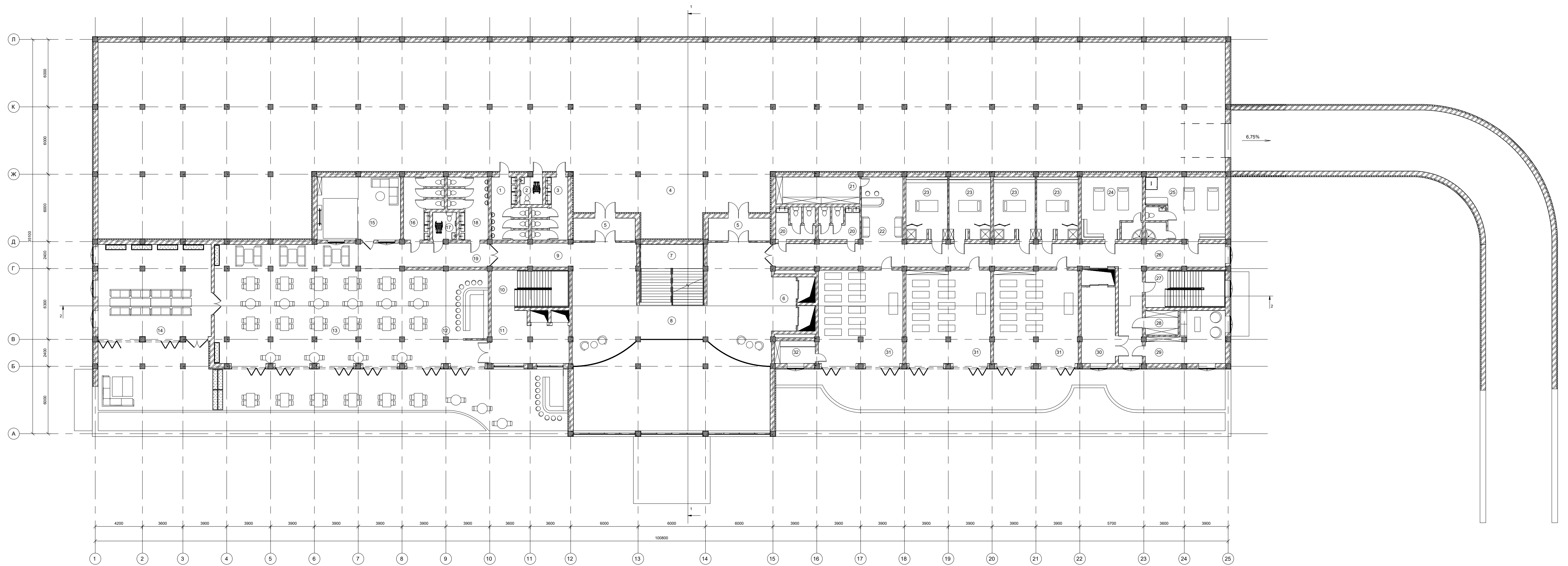
План на відмітці +3.600 М 1:200
