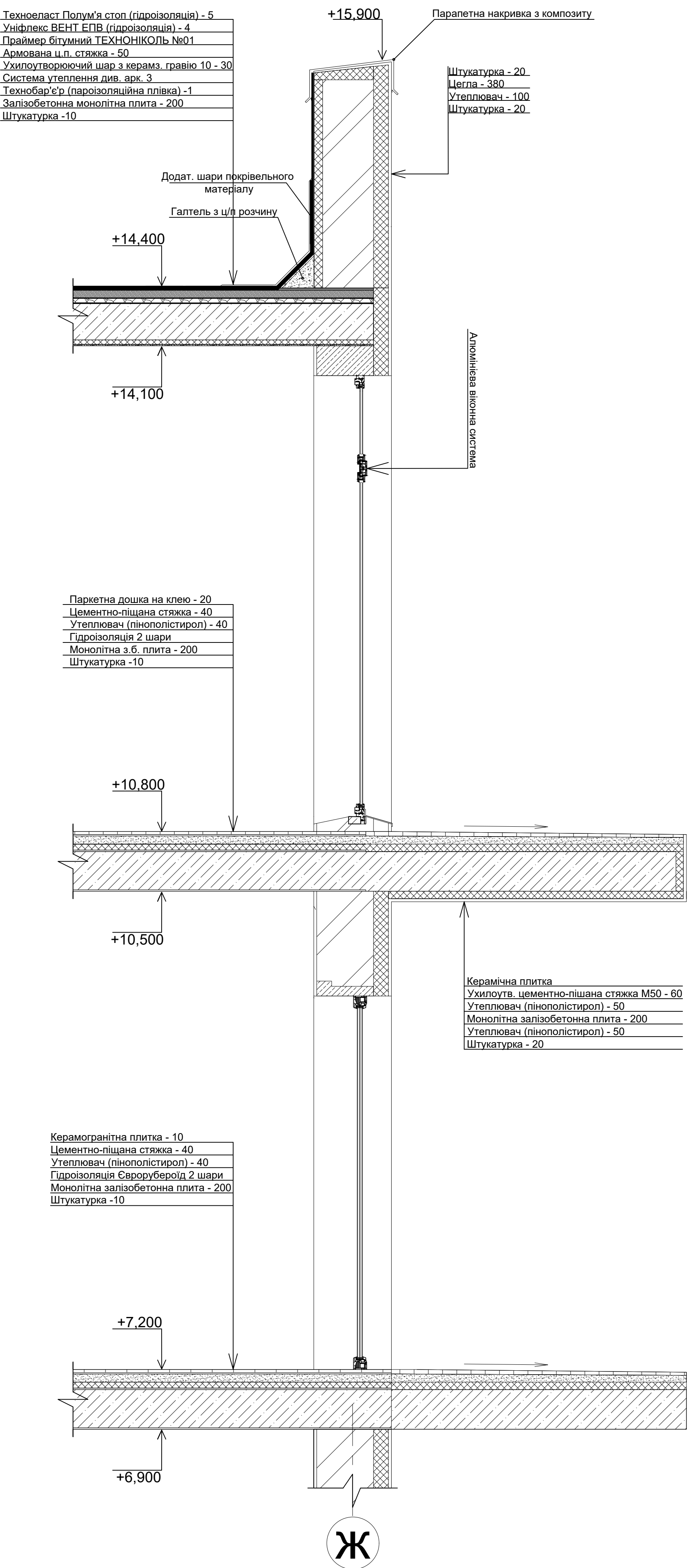
Розріз по стіні М 1:20
