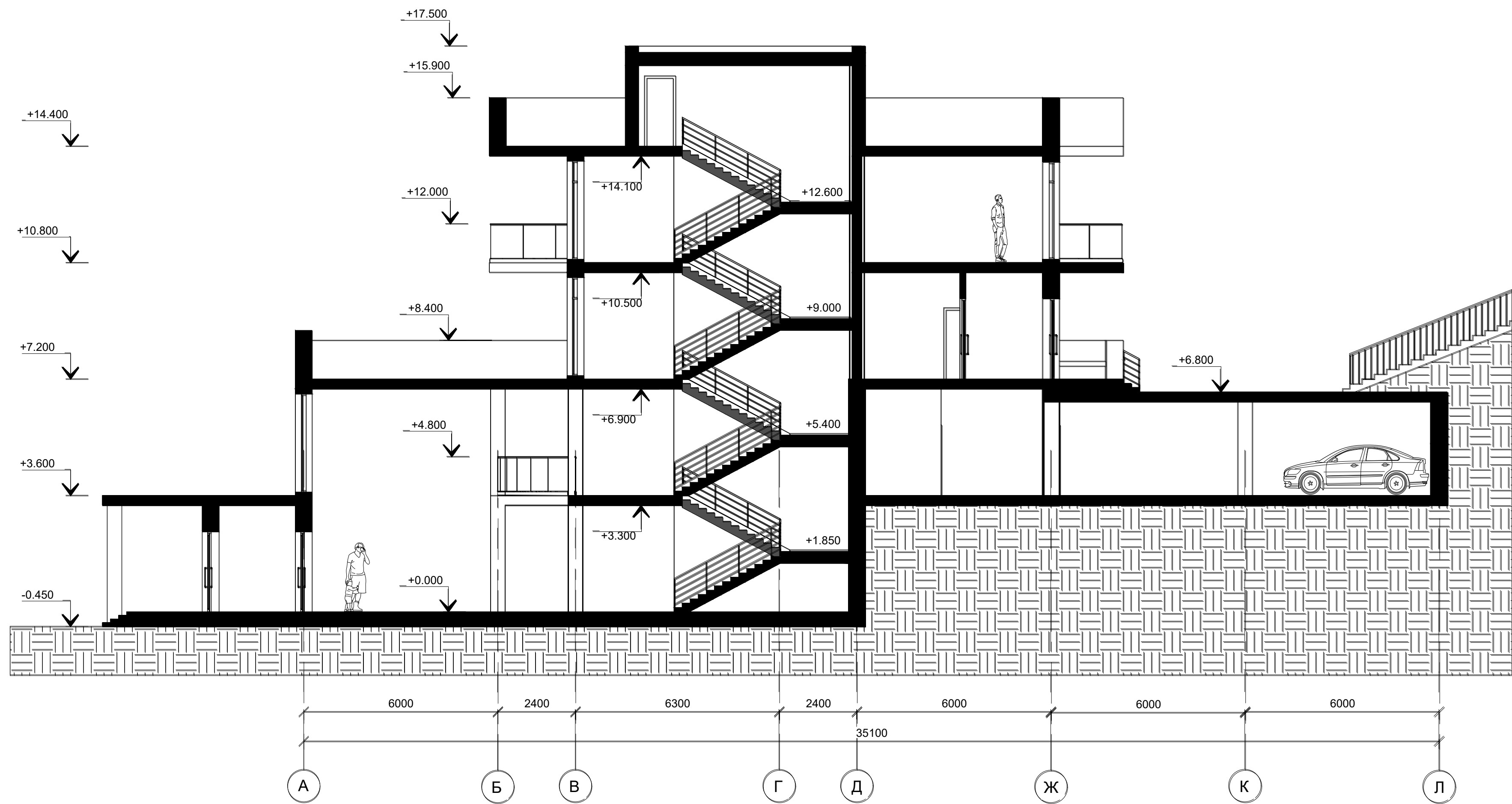
Розріз 1-1 М 1:100
