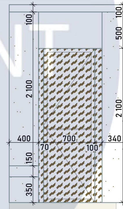
Розгортка санвузла 07 1:30
