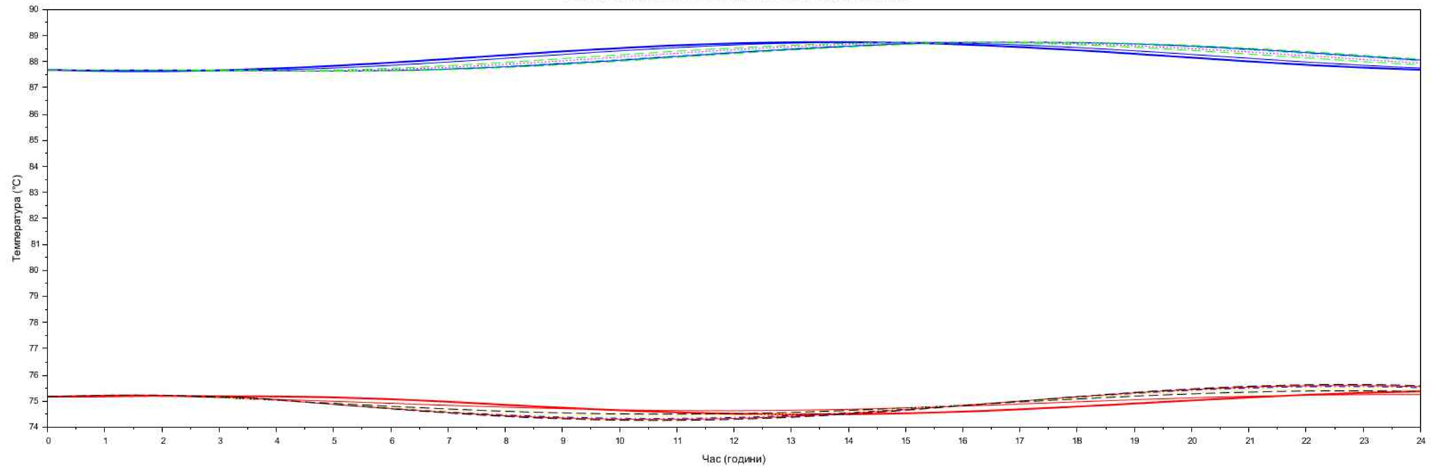
Температури подачі та зворотки в котельні та у споживачів
