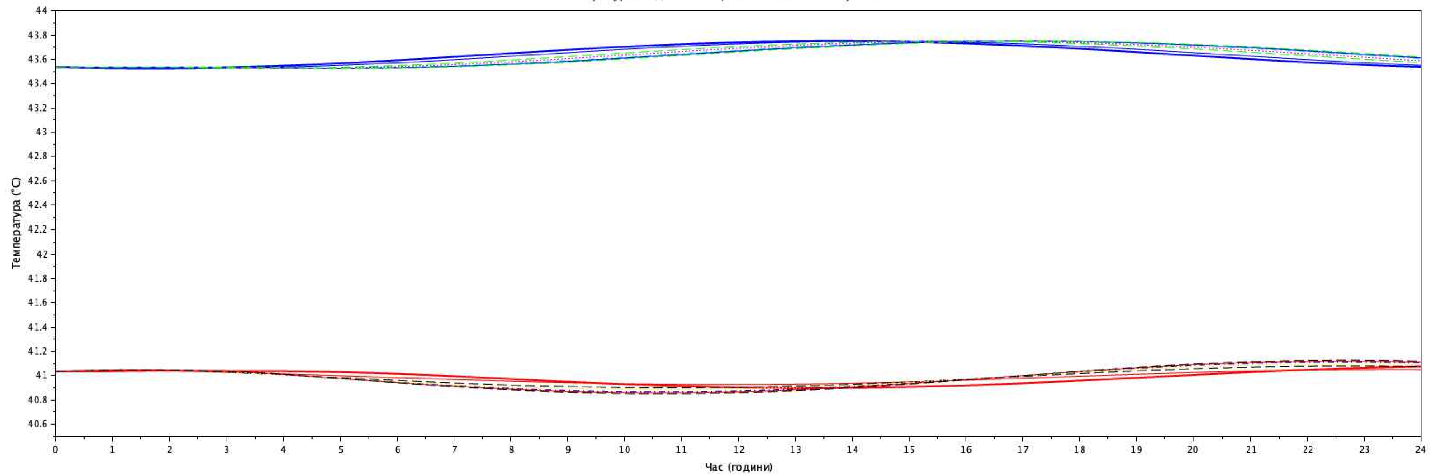
Температури подачі та зворотки в котельні та у споживачів
