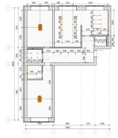
План стелі М 1:50
