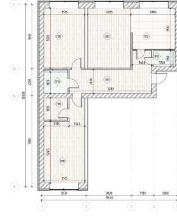
План підлоги М 1:50
