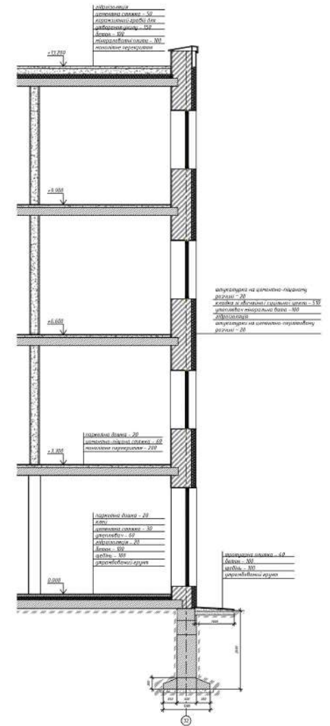
Розріз по стіні М 1:20
