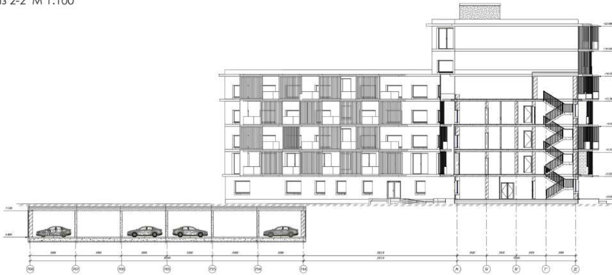
Розріз 1-1 М 1:100
