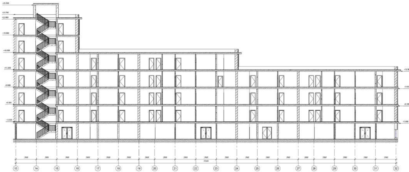
Розріз 2-2 М 1:100
