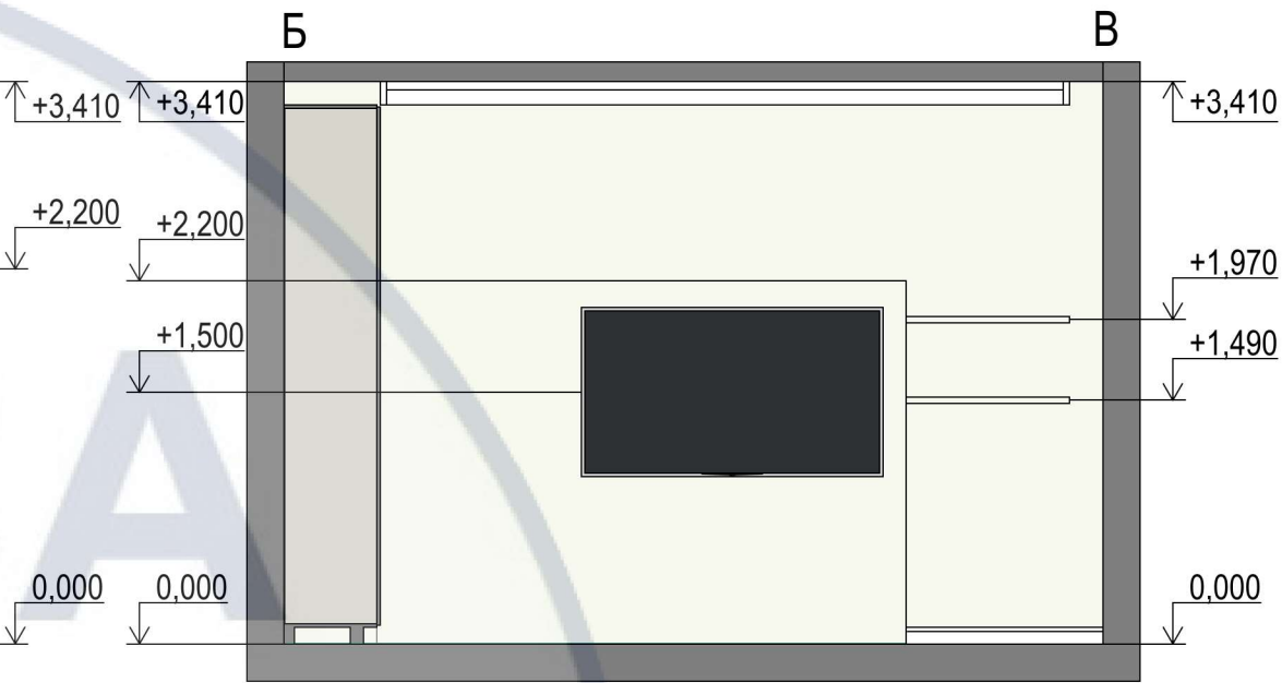
Розгортки БВ
