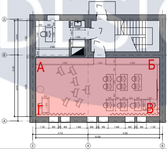
План приміщення М1:200
