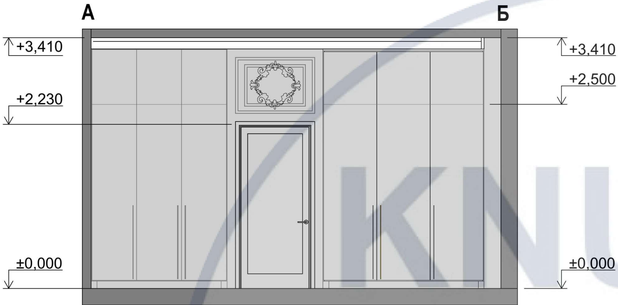
Розгортки АБ
