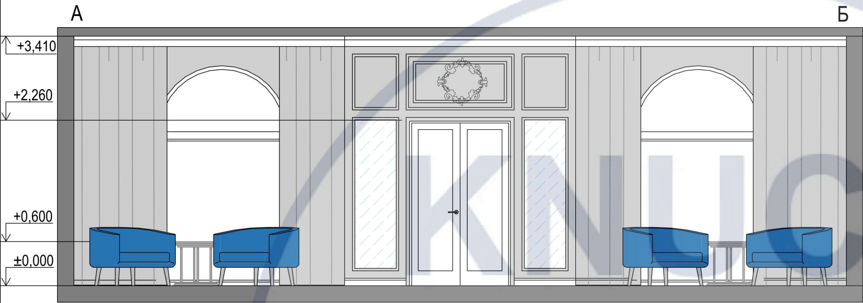
Розгортки АБ
