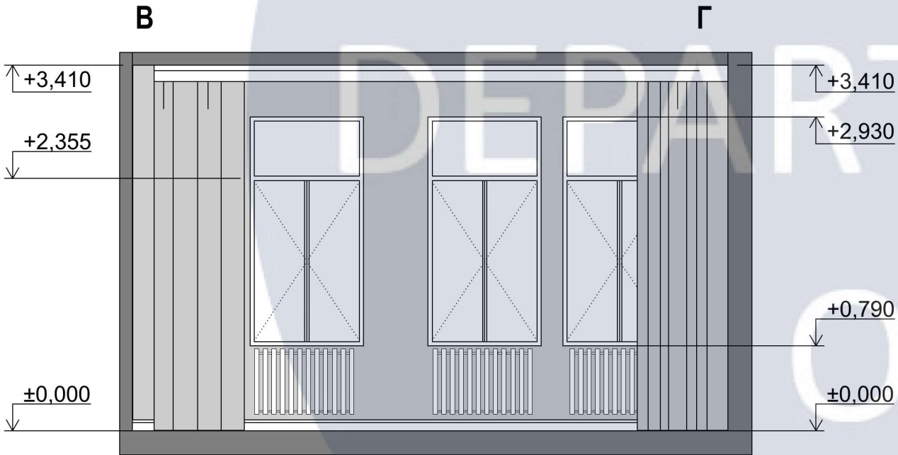
Розгортки ВГ
