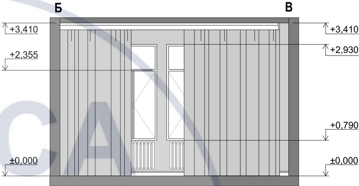
Розгортки БВ
