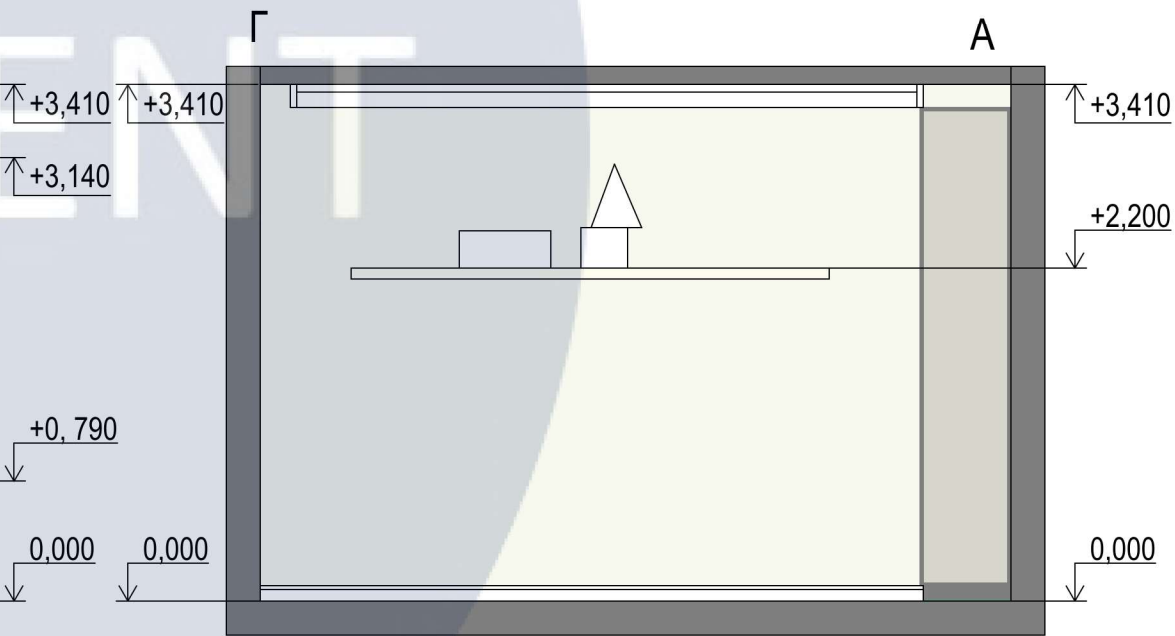
Розгортки ГА
