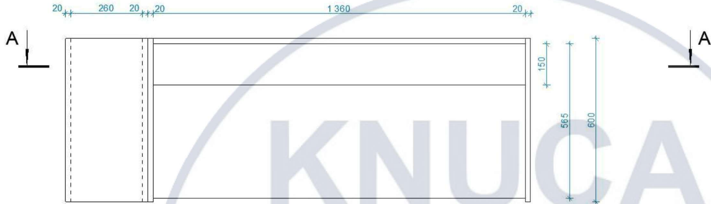
Вид спереду
