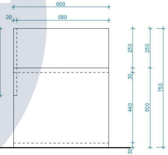
Вид збоку
