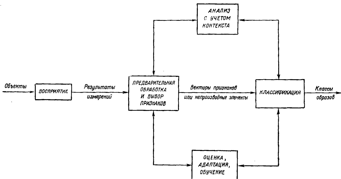
Рис. II-3. Схема адаптивної системи розпізнання образів (за Д. Ту та Р. Гонсалесом), що дозволяє паралельно виділяти класи на основі даної виборки та відносити об'єкти до них.
