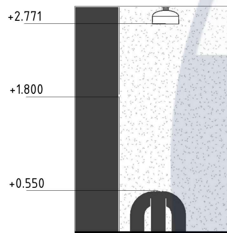
Розгортка 3-4 М 1:50
