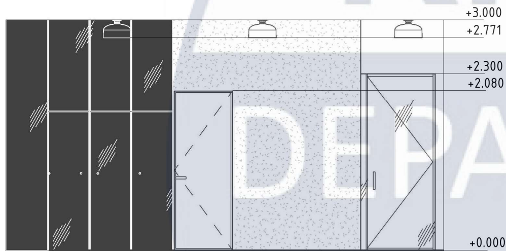
Розгортка 4-1 М 1:50
