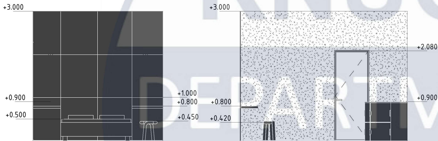
Розгортка 3-4 М 1:50
