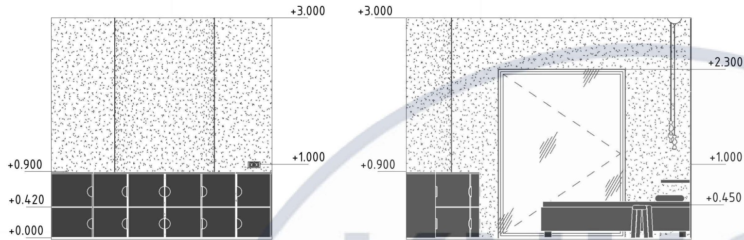
Розгортка 1-2 М 1:50
