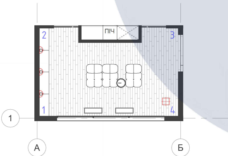
Планування вітальні М 1:75
