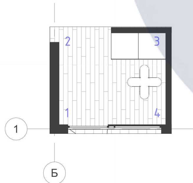
Планування тамбуру М 1:50
