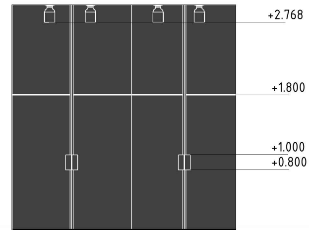
Розгортка 3-4 М 1:50
