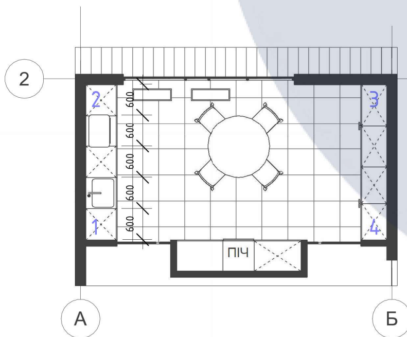
План кухні М 1:75
