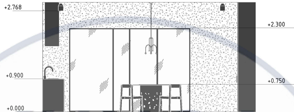
Розгортка 2-3 М 1:50
