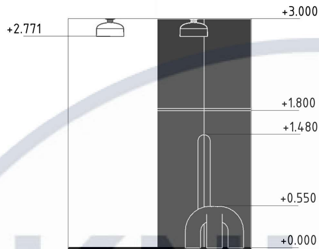
Розгортка 2-3 М 1:50
