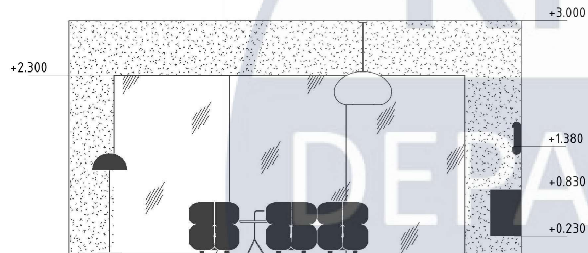
Розгортка 4-1 М 1:50
