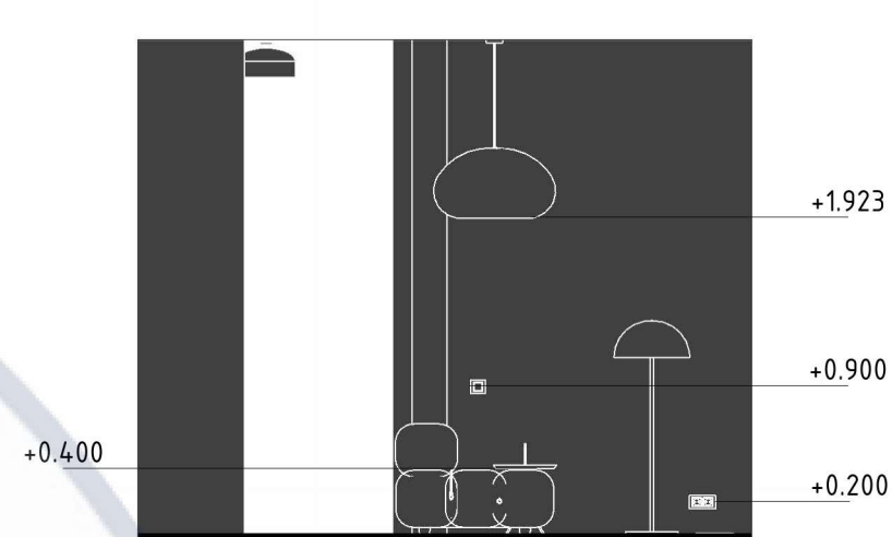
Розгортка 3-4 М 1:50
