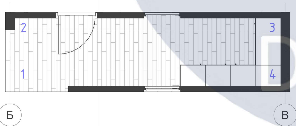
Планування коридору М 1:50
