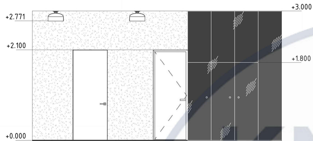
Розгортка 2-3 М 1:50
