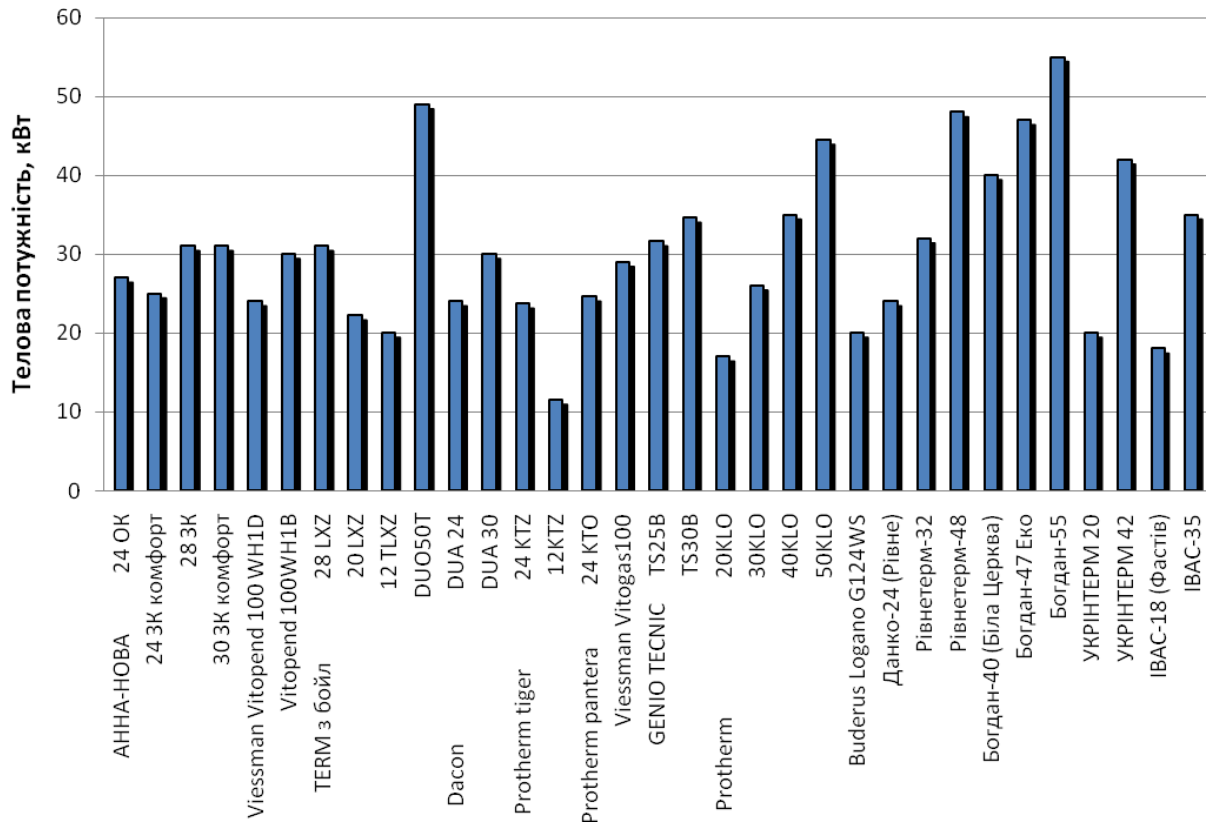
Рис. 1. Діаграма теплових потужностей котлів
