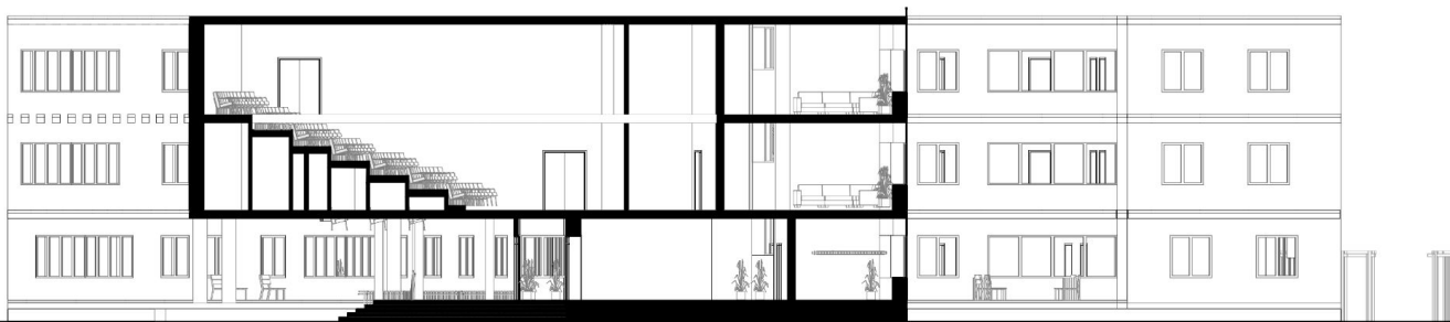
Розріз 2-2 М 1:100
