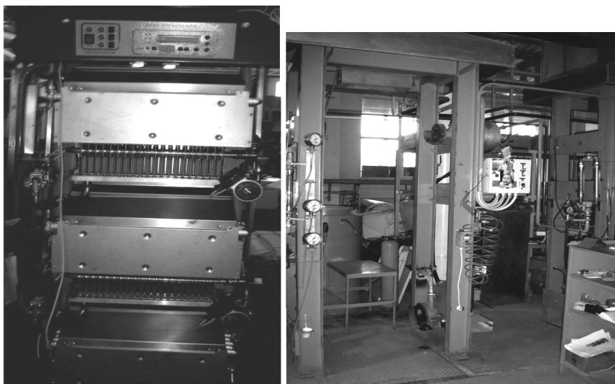
Рис. 4. Модуль нагріву МН ( a ) та лабораторний стенд для його випробування ( б )
