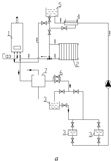
Рис. 1. Схема експериментального станда:
