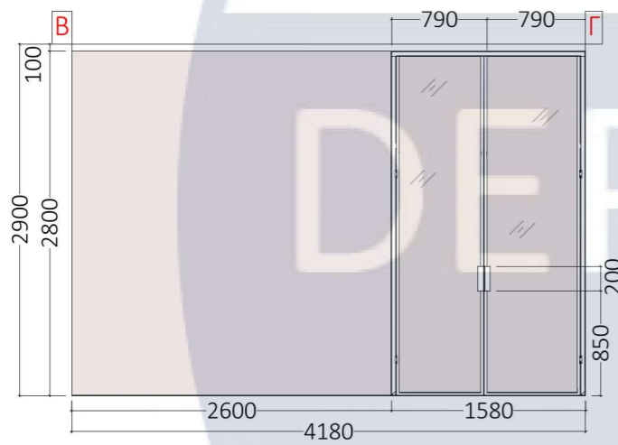
Розгортка В-Г
