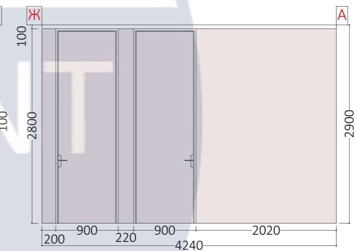
Розгортка Ж-А
