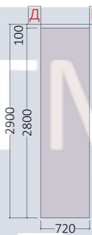
Розгортка Д-Е
