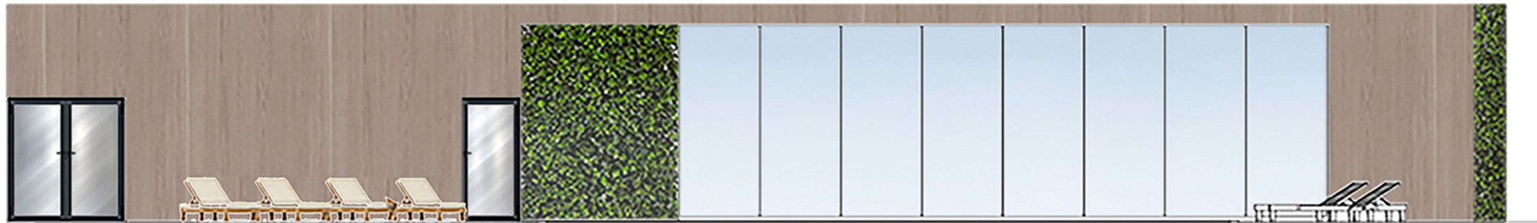
РОЗГОРТКА Г-Е М1:50
