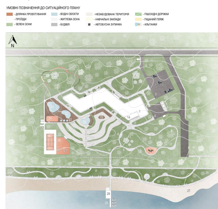
ГЕНЕРАЛЬНИЙ ПЛАН M1:500
