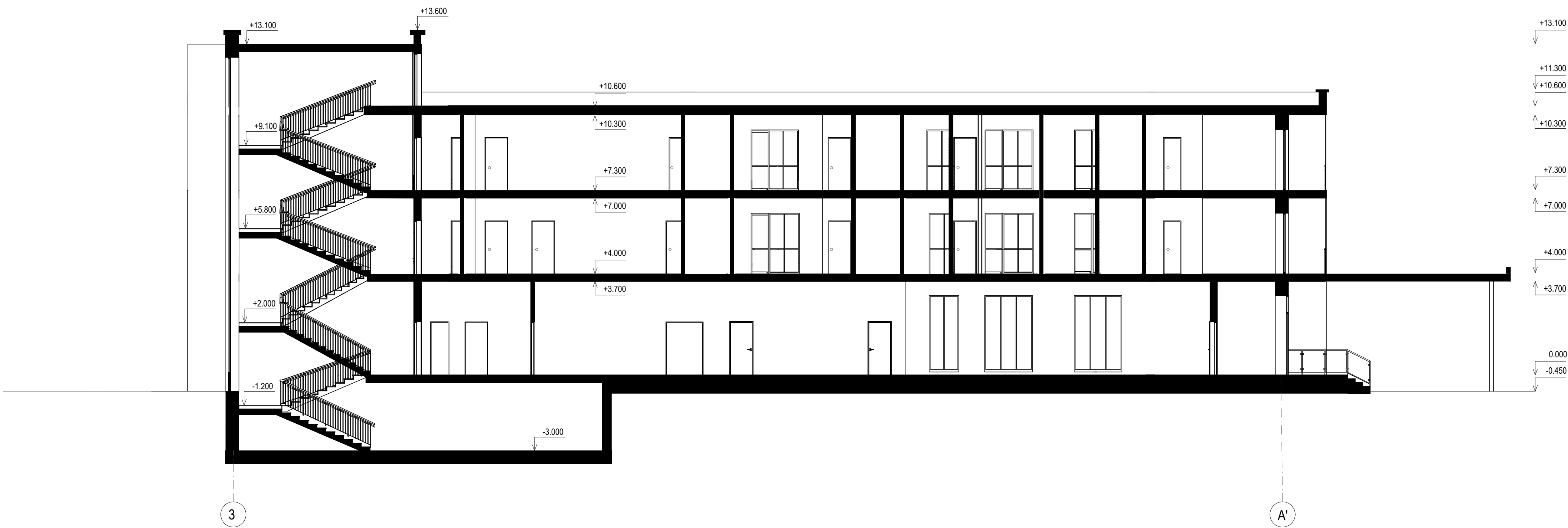
PO3PI3 2-2 M 1:100
