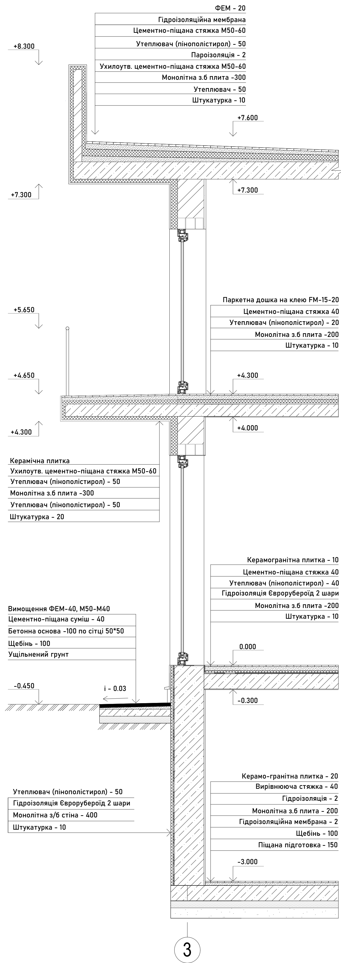
PO3PI3 3-3 M 1:25
