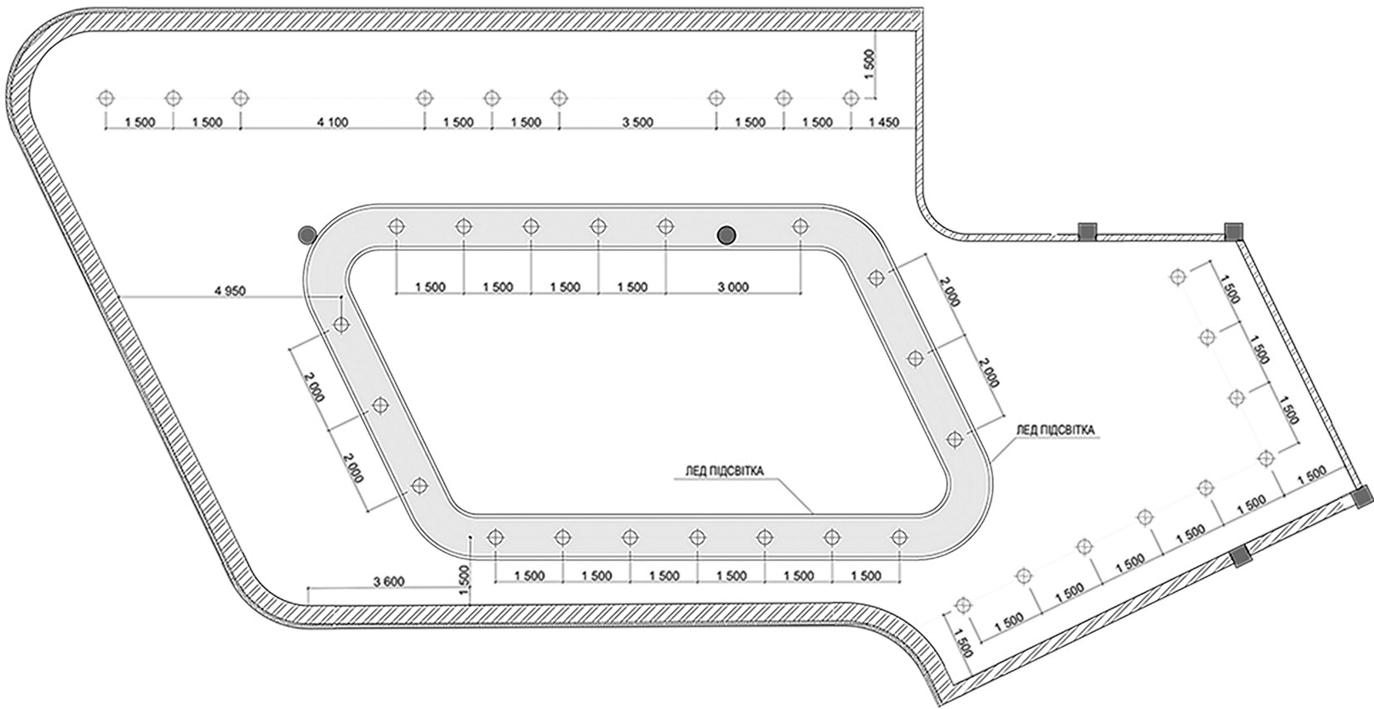
ПЛАН СТЕЛІ М1:50
