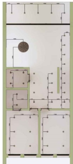
ПЛАН СТЕЛІ ДРУГОГО ПОВЕРХУ КВАРТИРИ М 1:50
