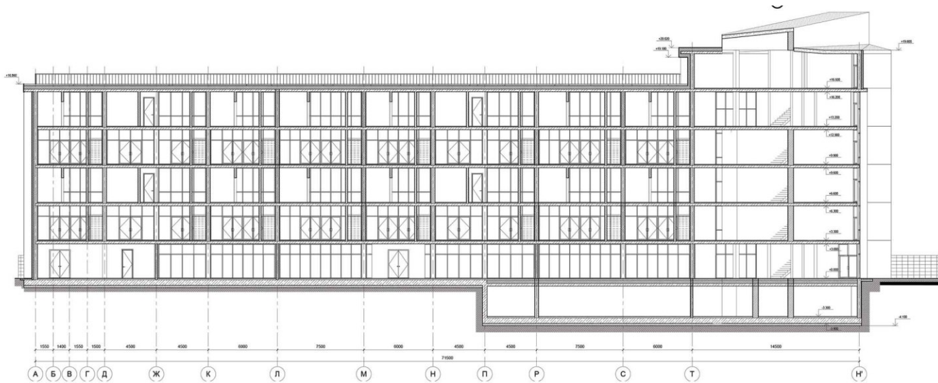
Розріз 2-2 М 1:200
