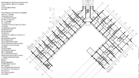
План третього поверху М 1:200
