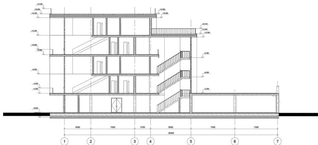
Розріз 2-2 М 1:200
