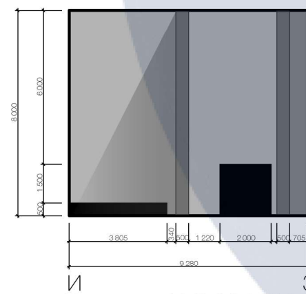
Розгортка І-З, М 1:200
