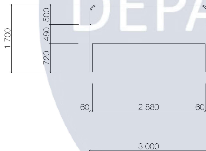
Вид зверху, М 1:50
