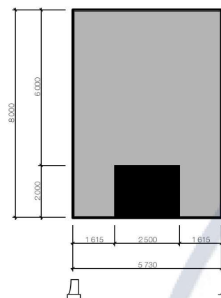
Розгортка Д-Л, М 1:200
