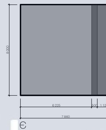
Розгортка Є-Е, М 1:200
