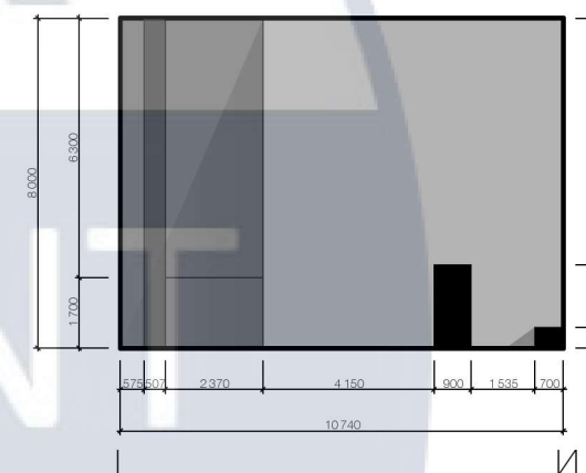
Розгортка І-І, М 1:200
