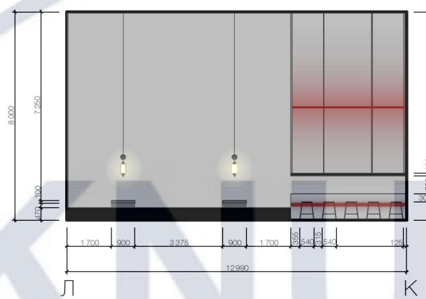
Розгортка Л-К, М 1:200
