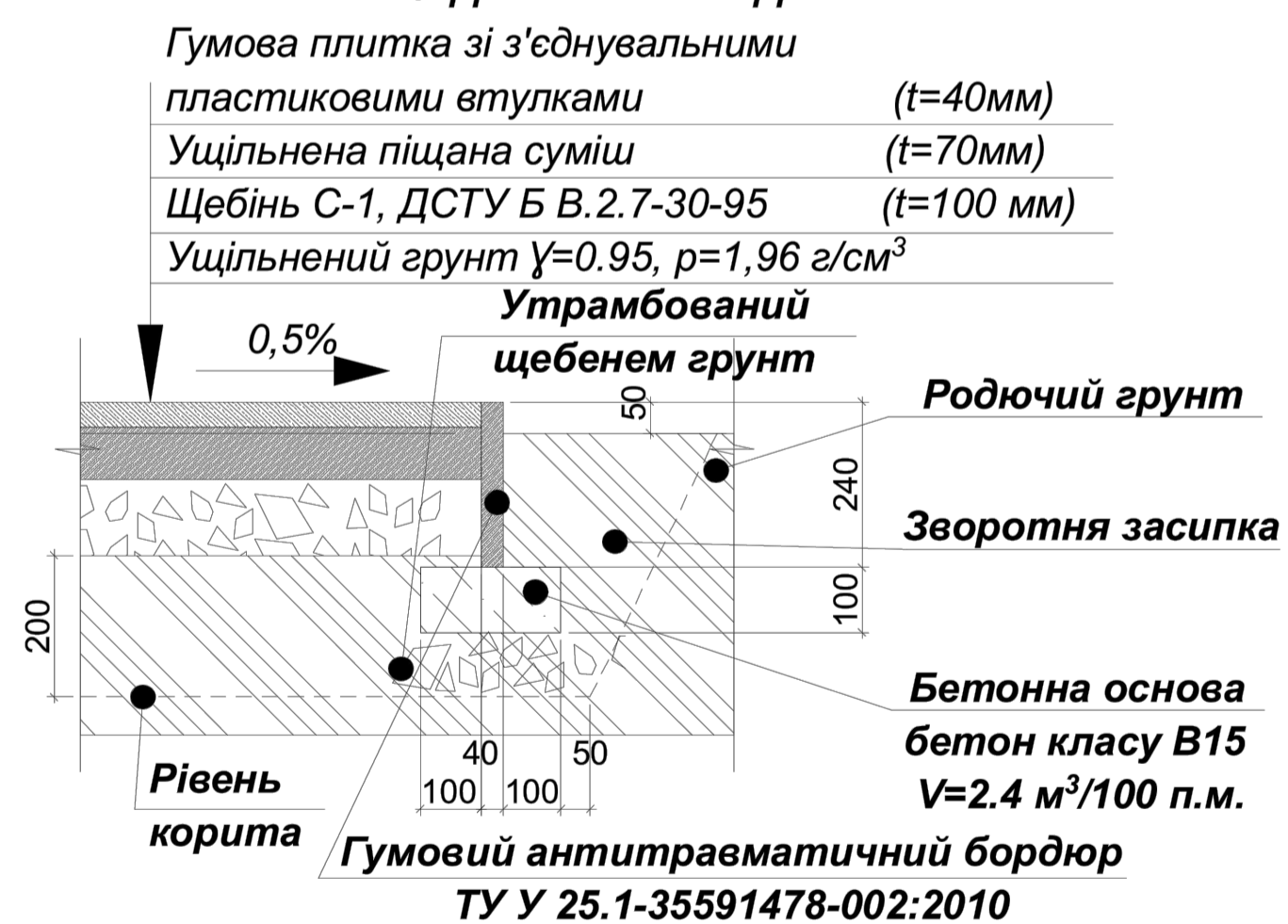
ТИП 3. ДИТЯЧИЙ МАЙДАНЧИК
