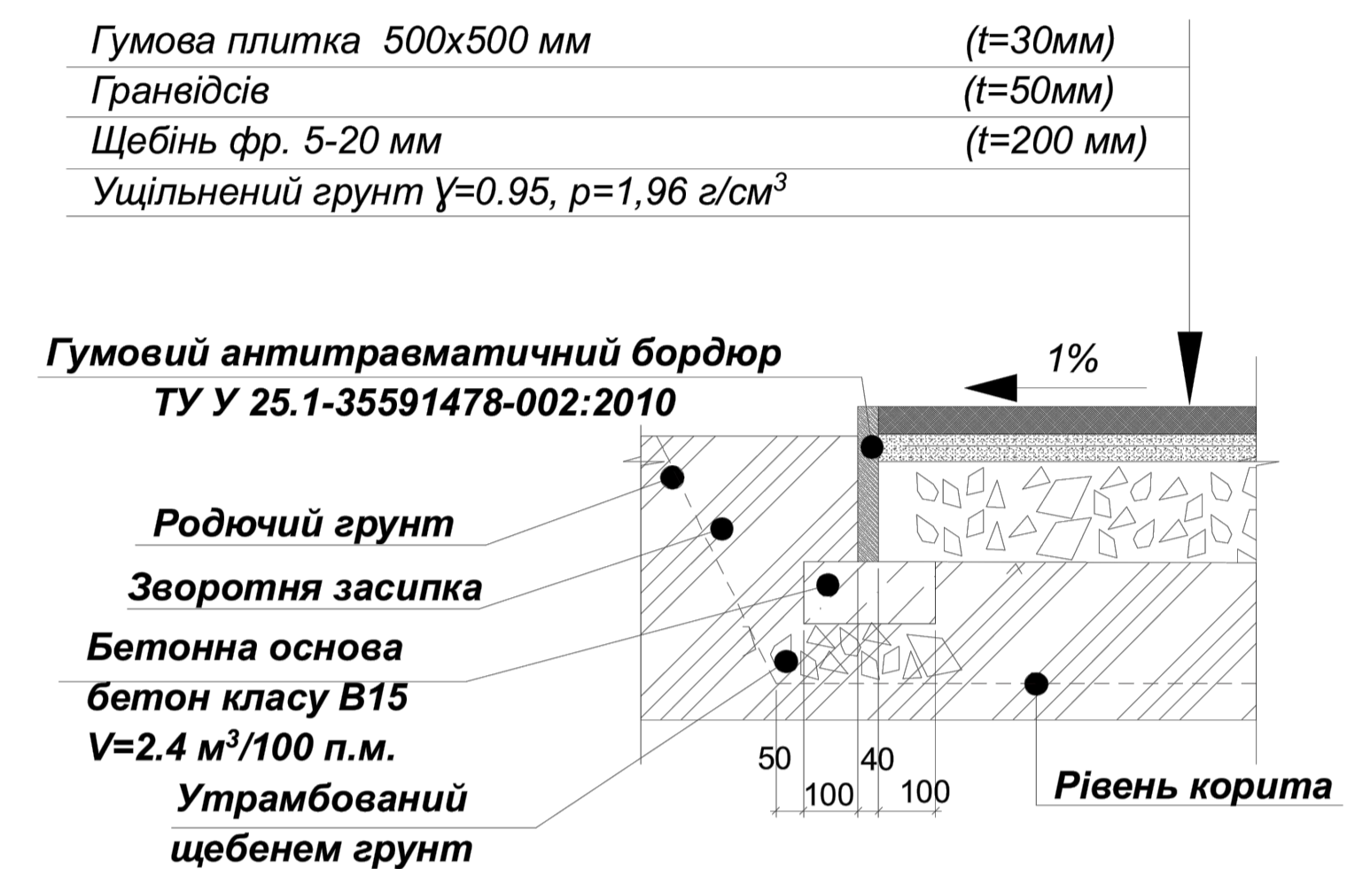
ТИП 2. ПОКРИТТЯ СПОРТИВНОГО МАЙДАНЧИКА
