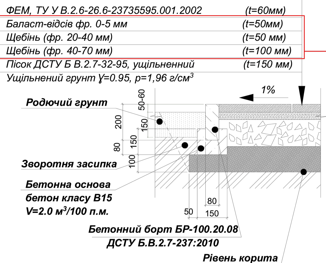
ТИП 1. ПОКРИТТЯ ТРОТУАРУ
