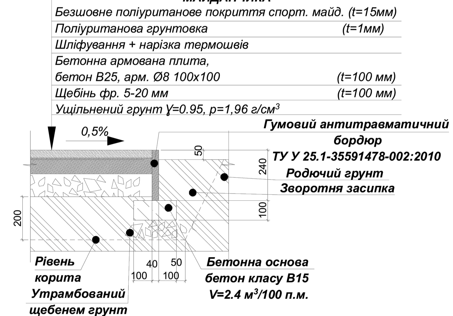
ТИП 4. ПОКРИТТЯ УНІВЕРСАЛЬНОГО СПОРТИВНОГО МАЙДАНЧИКА
