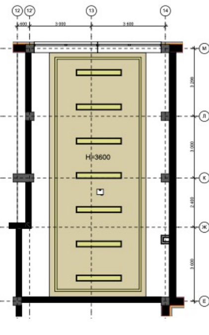
План стелі на відмітці 3,600 м
