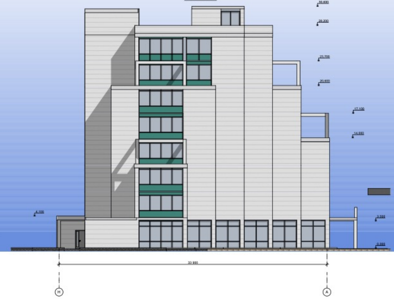
Фасад Н-А
