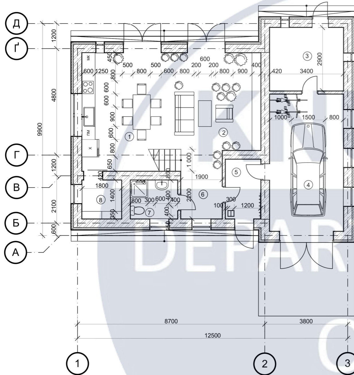
Експлікація приміщень першого поверху
