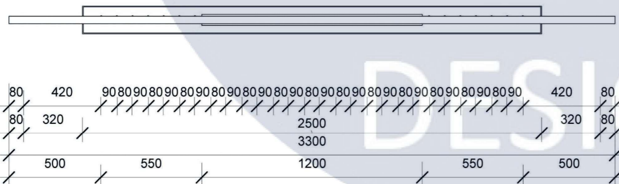
Вид зверху М 1:20
