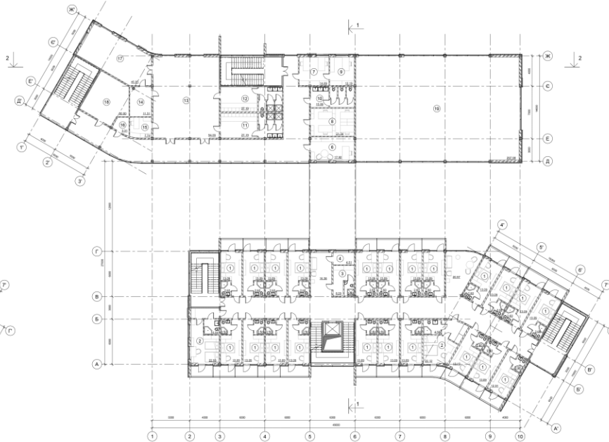
План поверху на відмітці +4,300 М1:200
