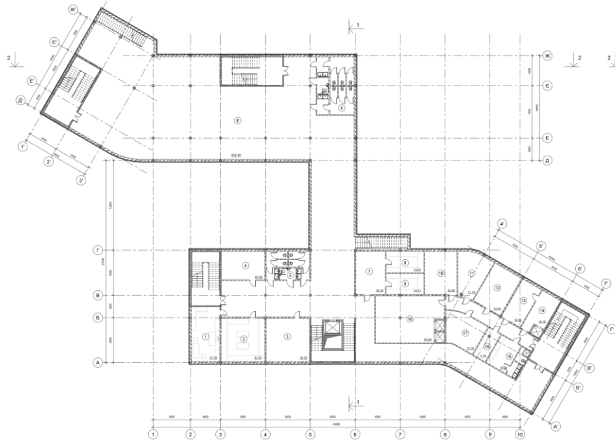
План поверху на відмітці -3,750 М1:200
