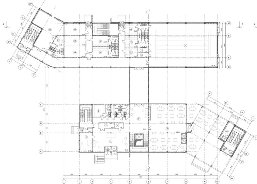
План поверху на відмітці +0,000 М1:200
