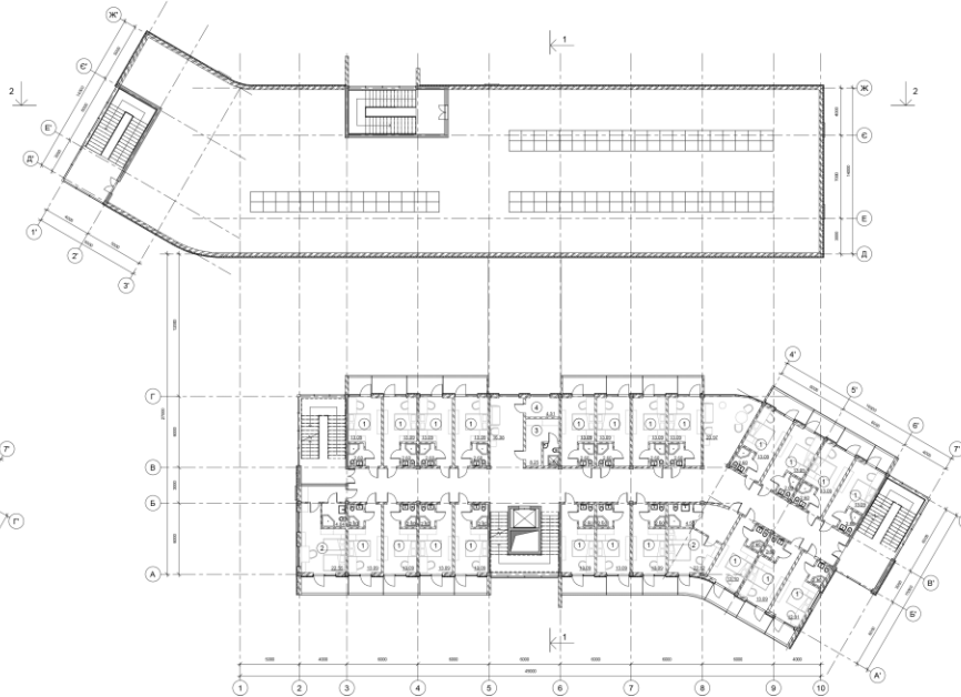
План поверху на відмітці +7,900 М1:200
