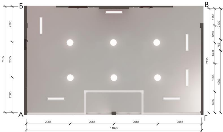
План стелі з освітлювальними приладами М1:50
