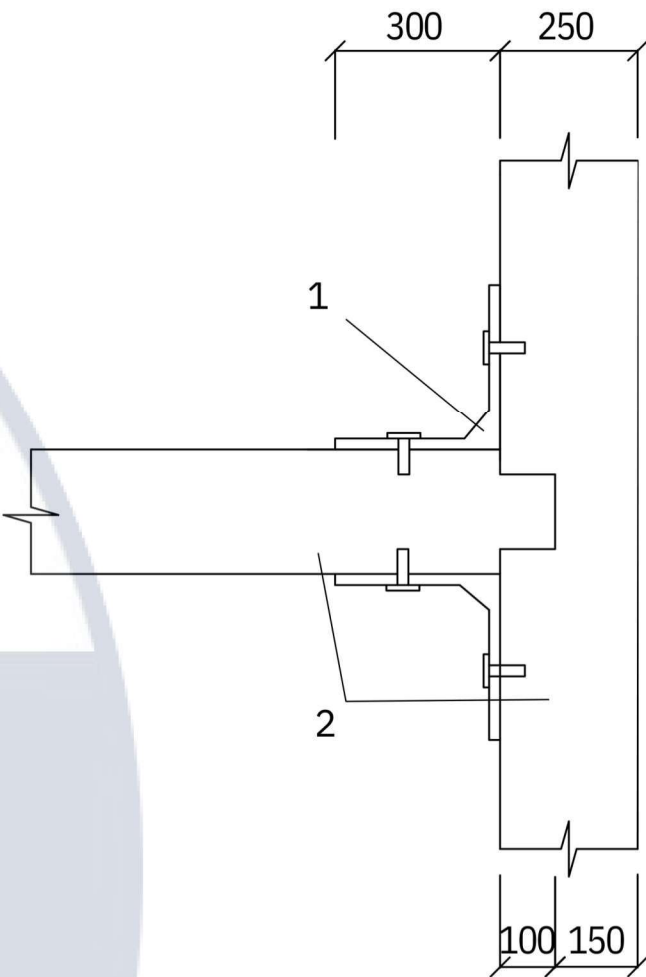
Вузол 1 М 1:2
