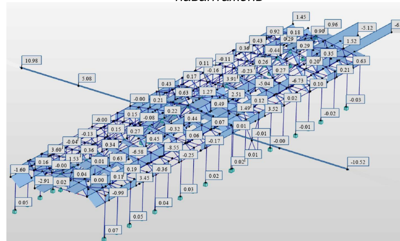
Зусилля Fy перевірного розрахунку від навантажень
