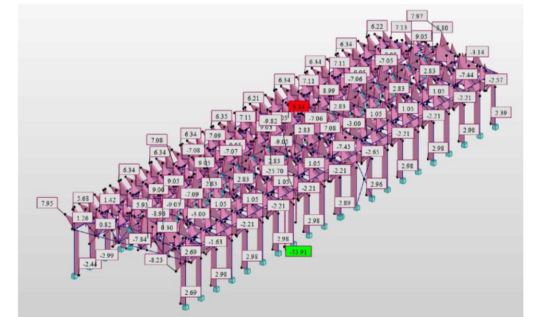
Зусилля Fz перевірного розрахунку від комбінацій навантажень
