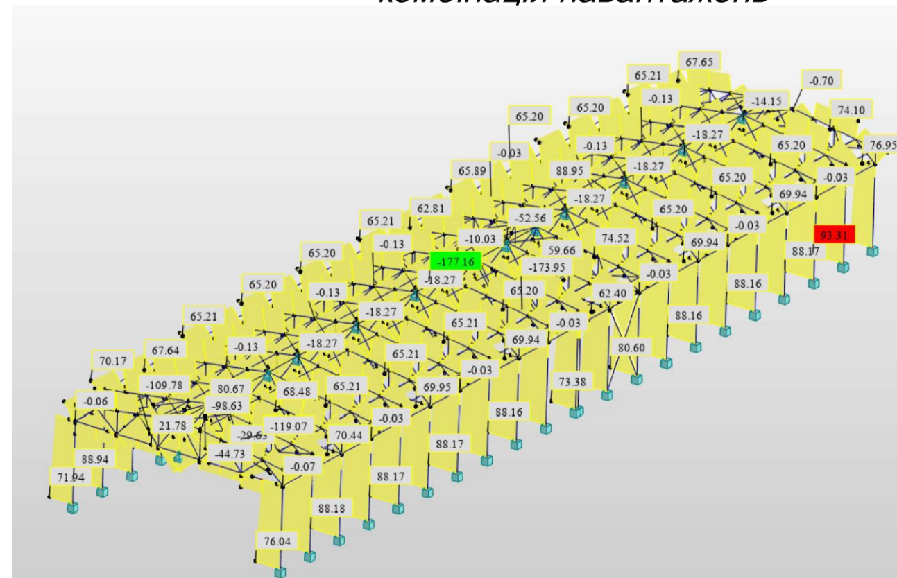
Зусилля Fx перевірного розрахунку від комбінацій навантажень
