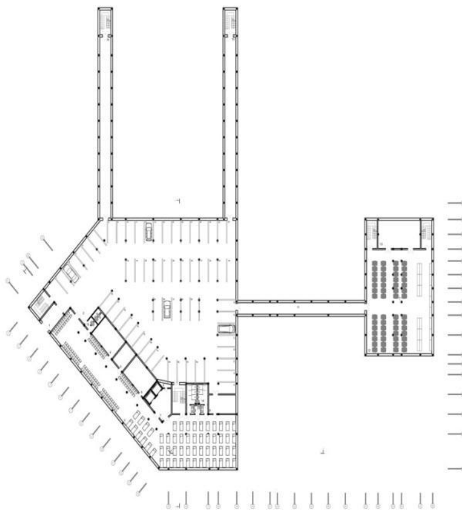
План підвального поверху М 1:400
