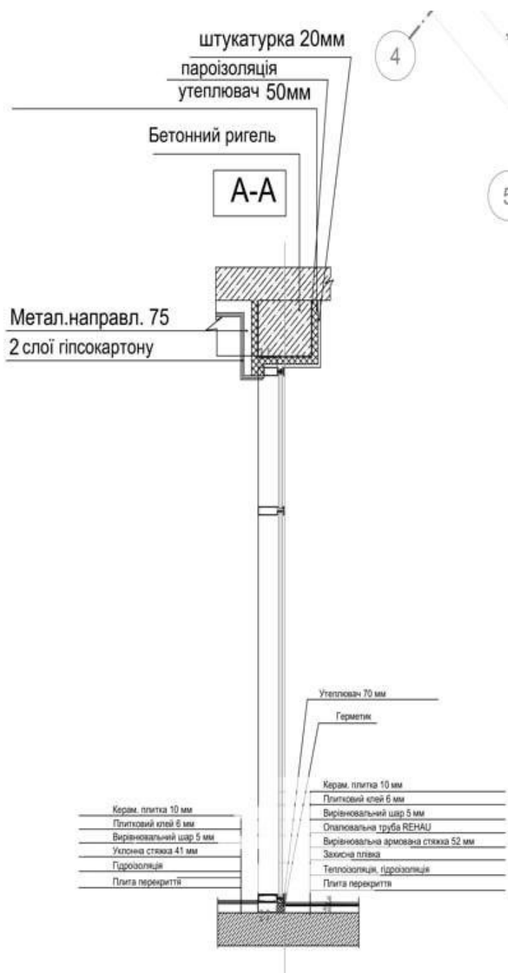
Рис.6.3 Розріз по стіні
