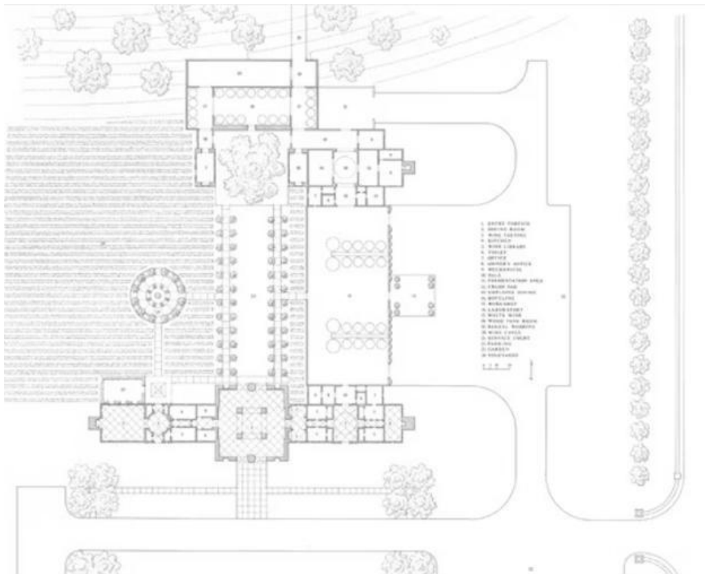
Рис. 2.6,7 Вигляд будівлі, Генеральний план [4]
