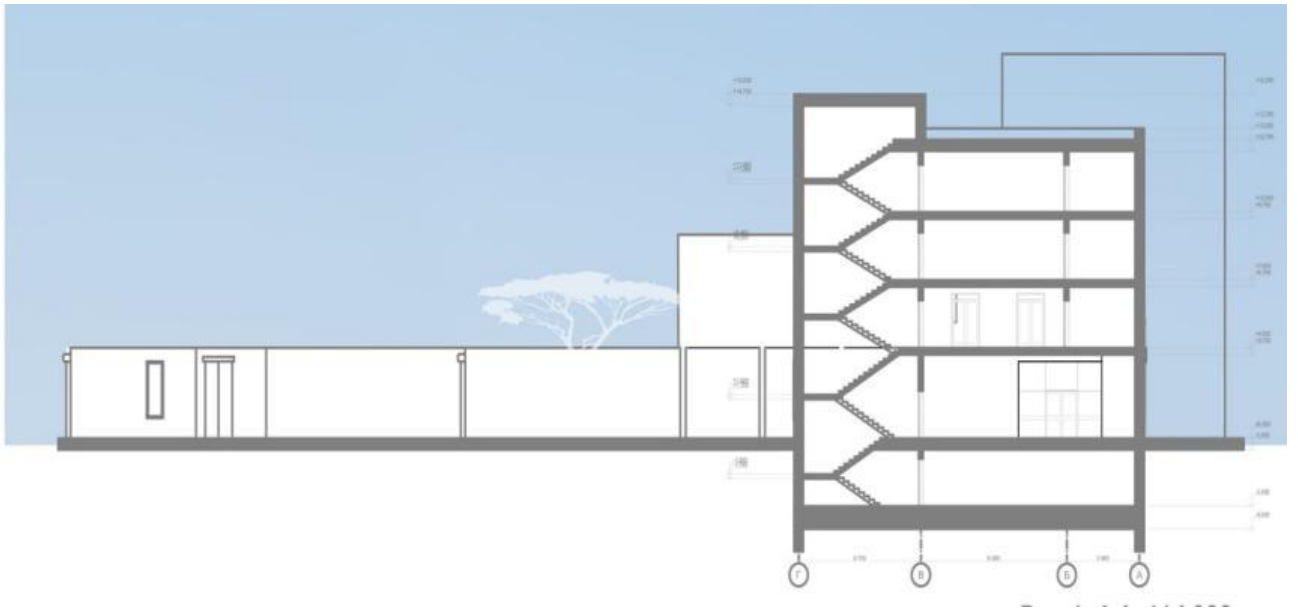
Розріз 2-2
