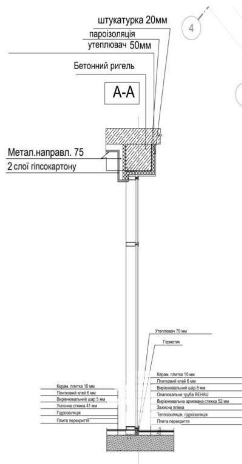
Розріз постіні
