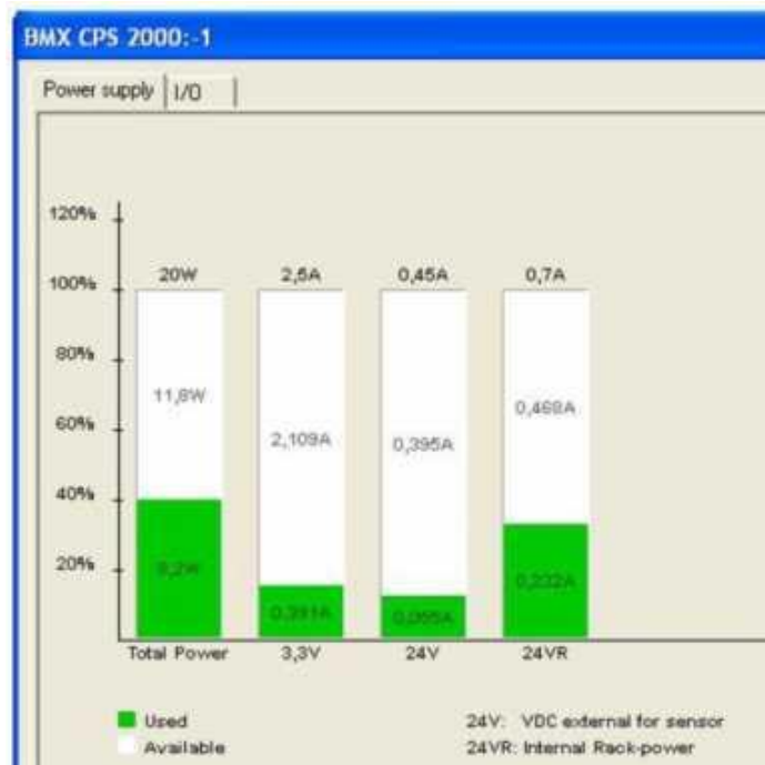
Рис. 7. Вікно розподілу споживаної потужності
