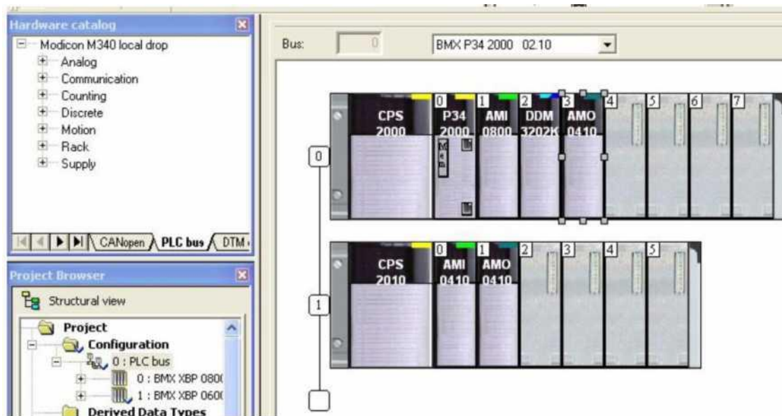
Рис. 4 . Вікно апаратної конфігурації
