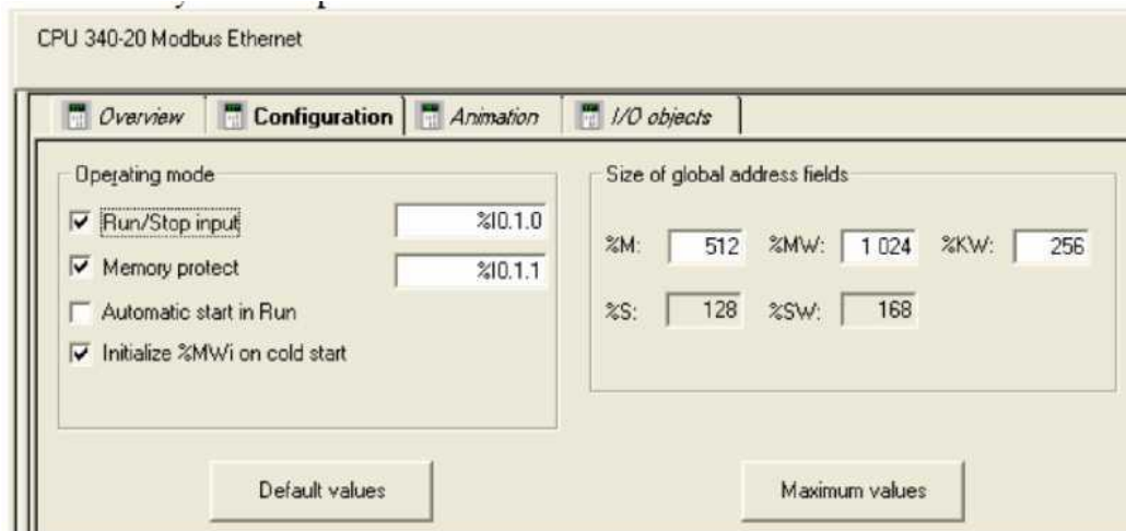
Рис. 6. Вікно конфігурації процесорного модуля
