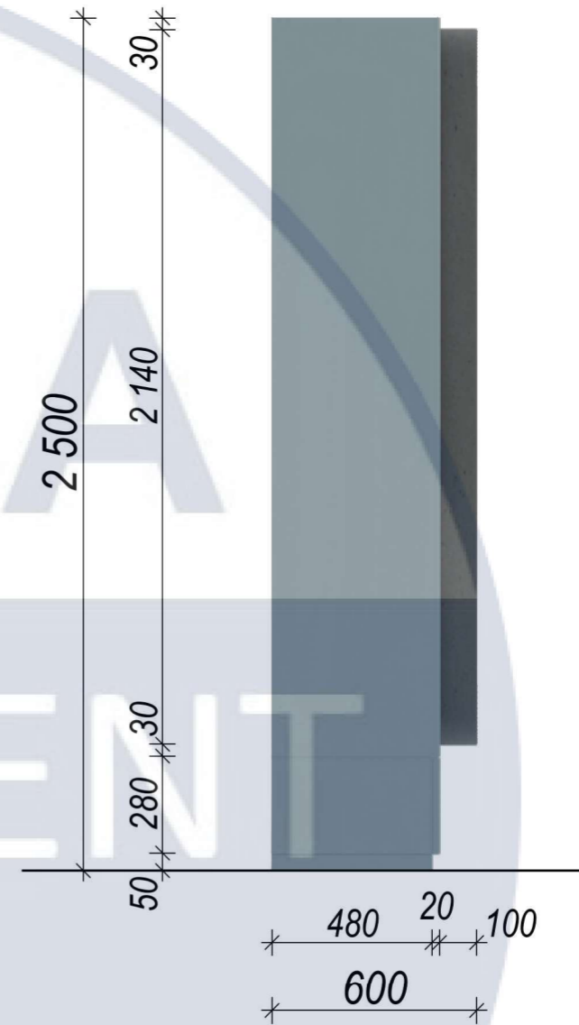
Вид збоку, М 1:20
