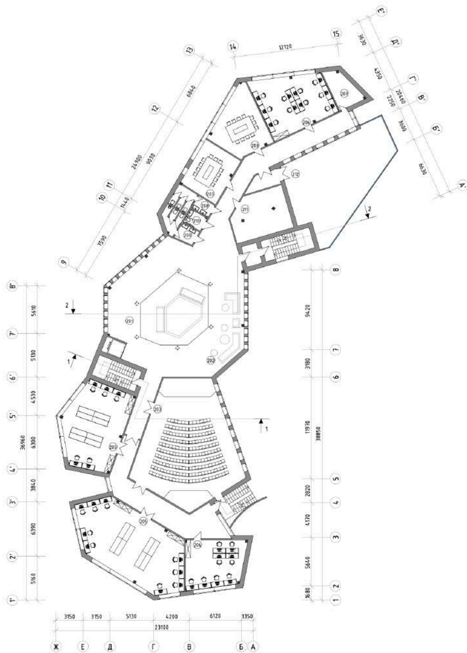
Рис. 4.2. План поверху на відмітці +3.600
