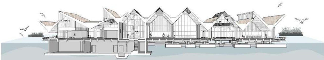
Рис. 2.33 «Wetland Research and Education Center», Розріз будівлі. [13]
