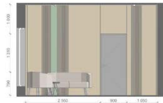
Розгортка Б-В М1:50
