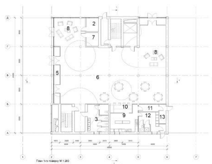
План 1-го поверху М 1:200
