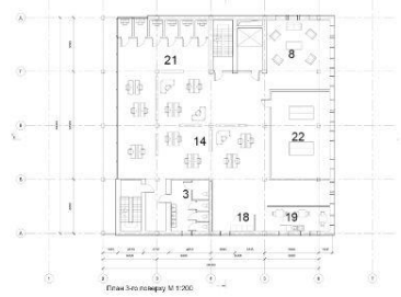
План 3-го поверху М 1:200
