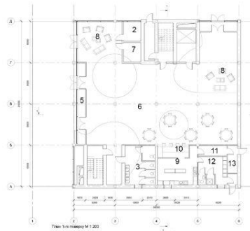
План 1-го поверху М 1:200
