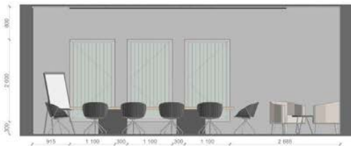
Розгортка В-Г М1:50
