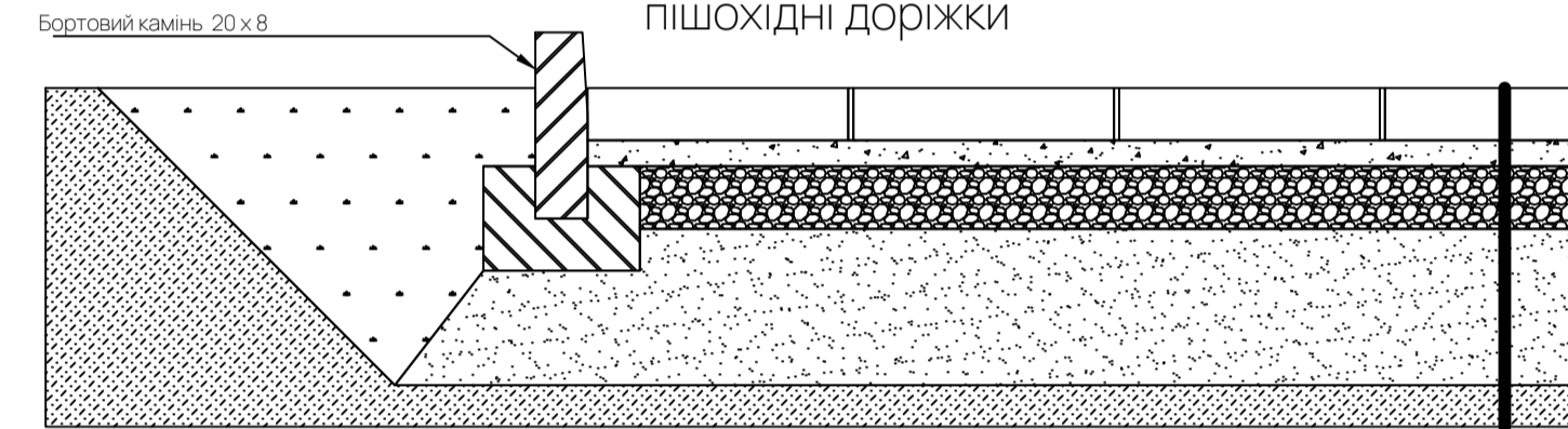
Конструкція плиточного покриття пішохідні доріжки
