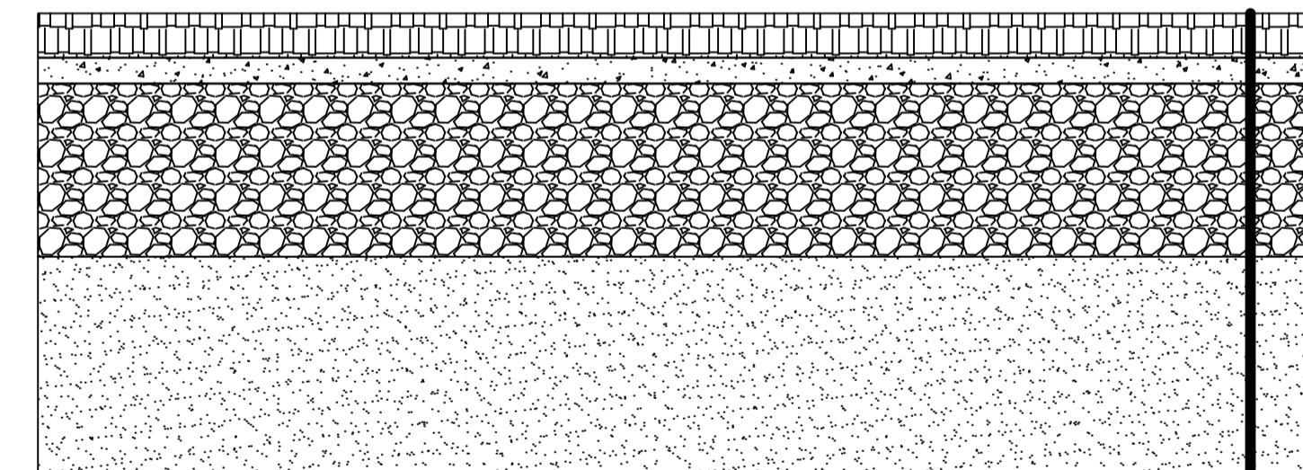
Конструкція покриття паркінгу
