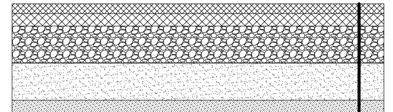
Конструкція асфальтобетонного покриття
