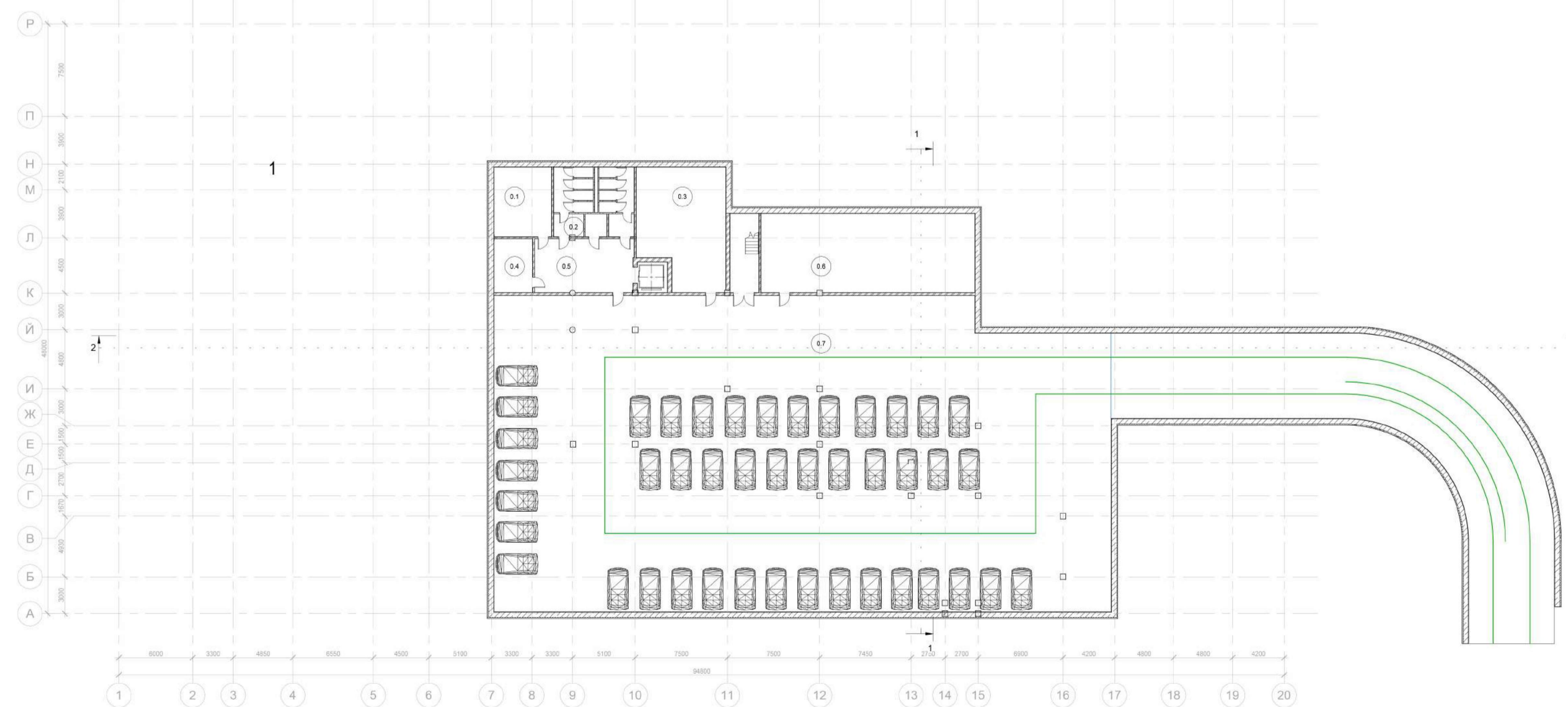
План підземного поверху M200
