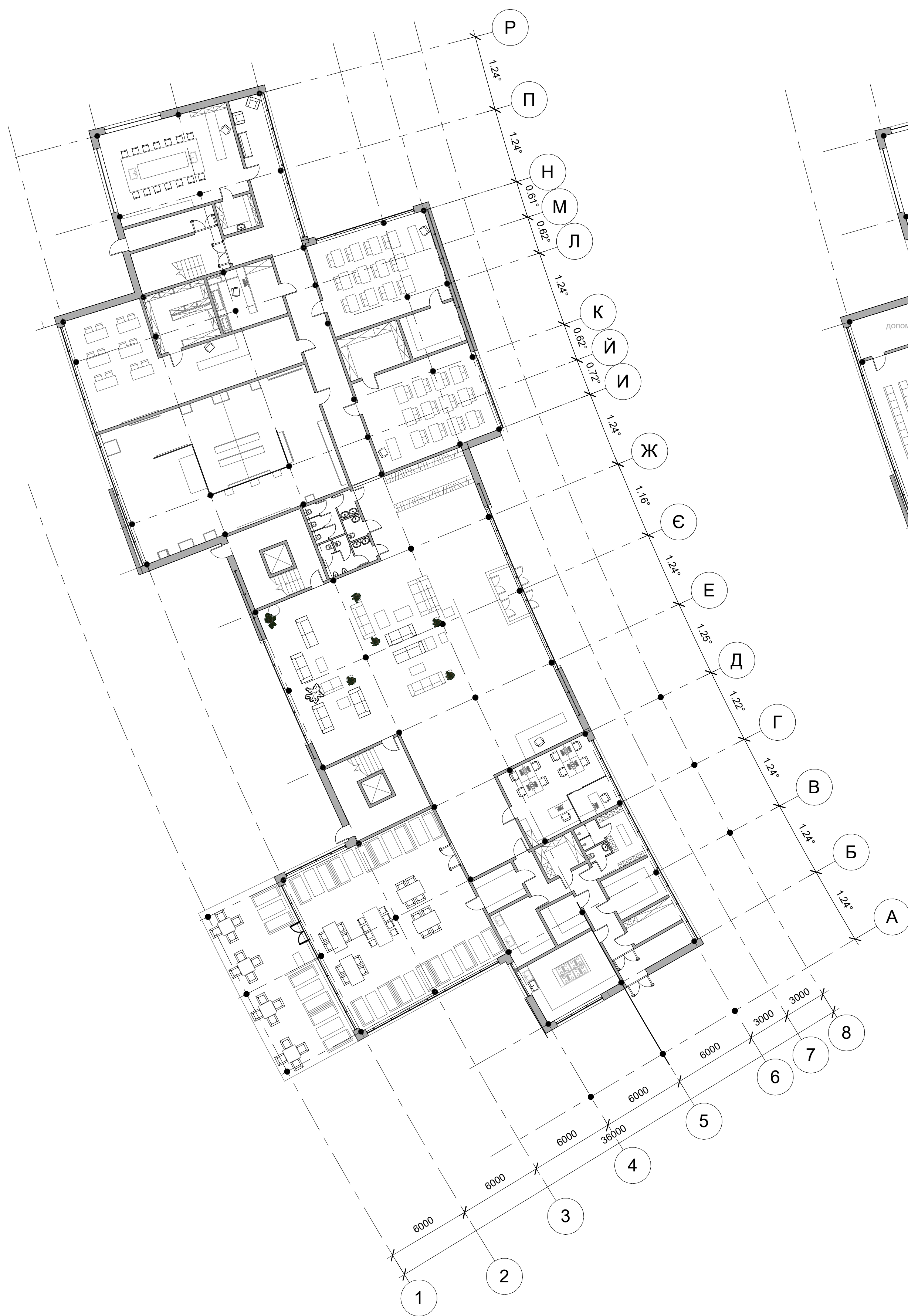
План на відмітці +0.000
