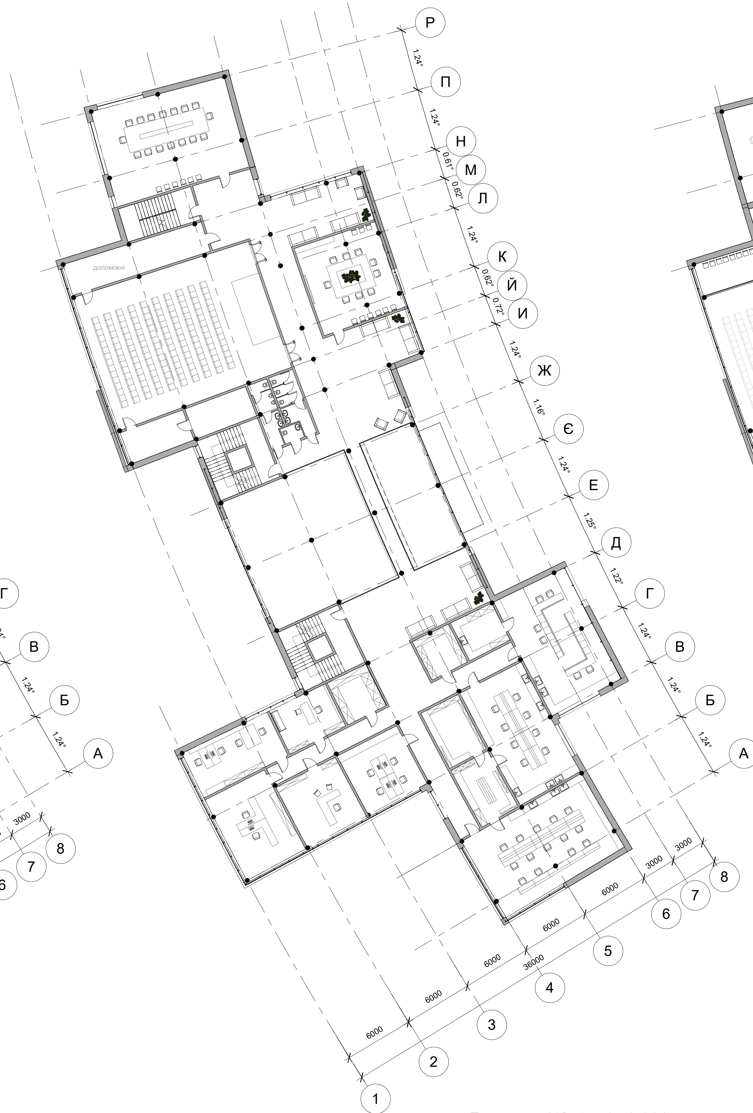
План на відмітці +0.000
