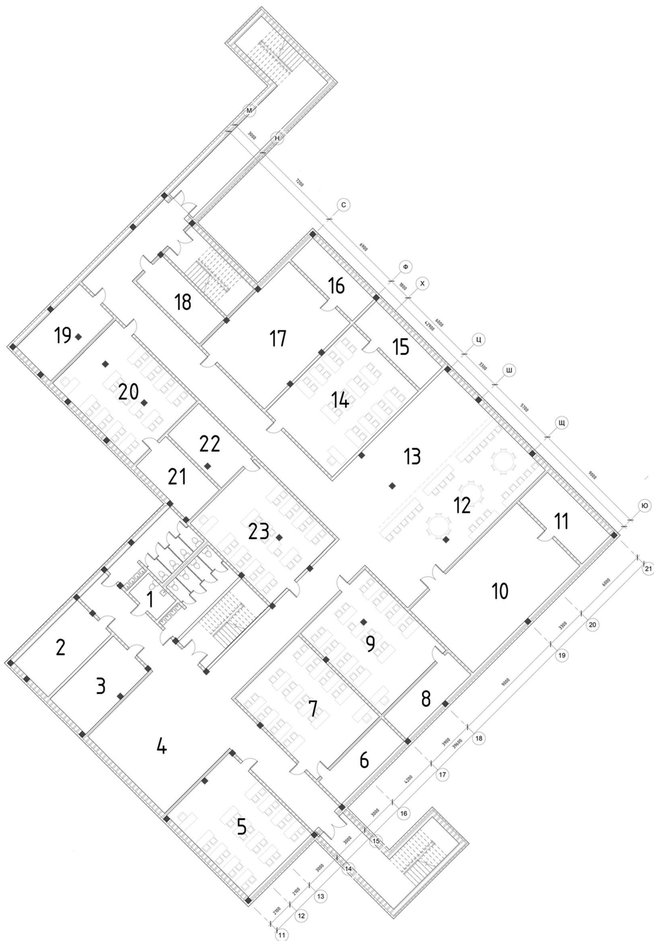
ПЛАН НА ВІДМІТЦІ -3.600 М 1:200
