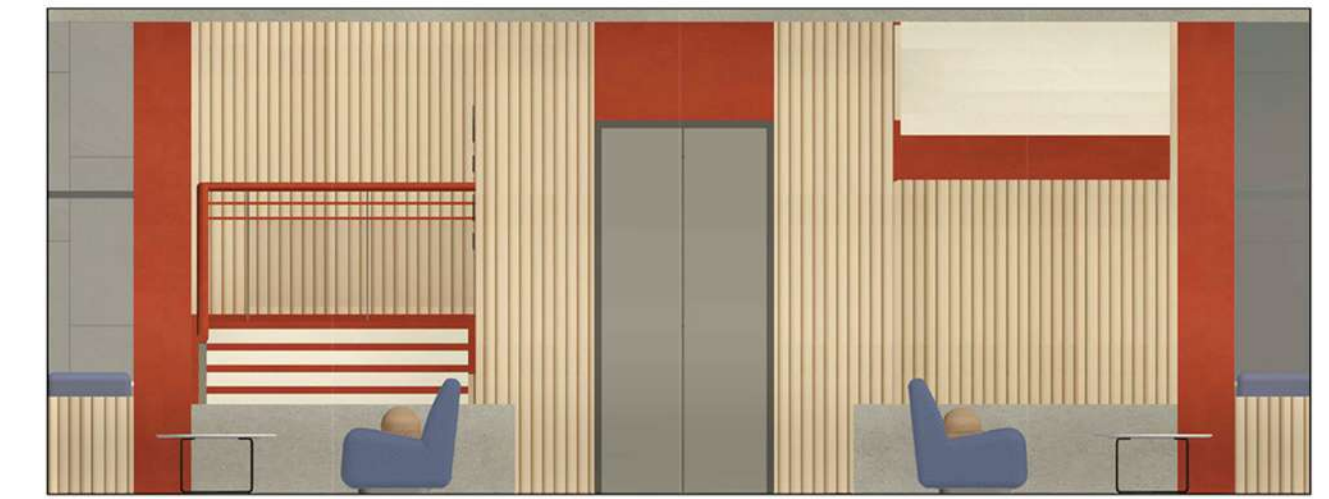
ВИД 4 М 1:50
