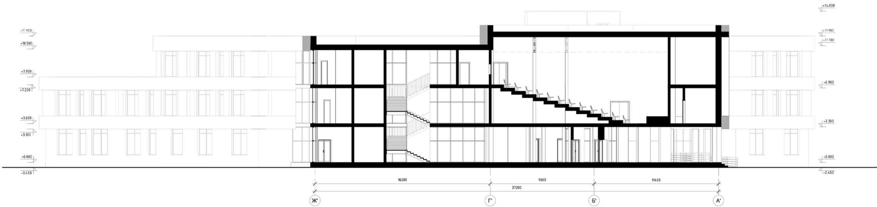
РОЗРІЗ 1-1 М 1:200
