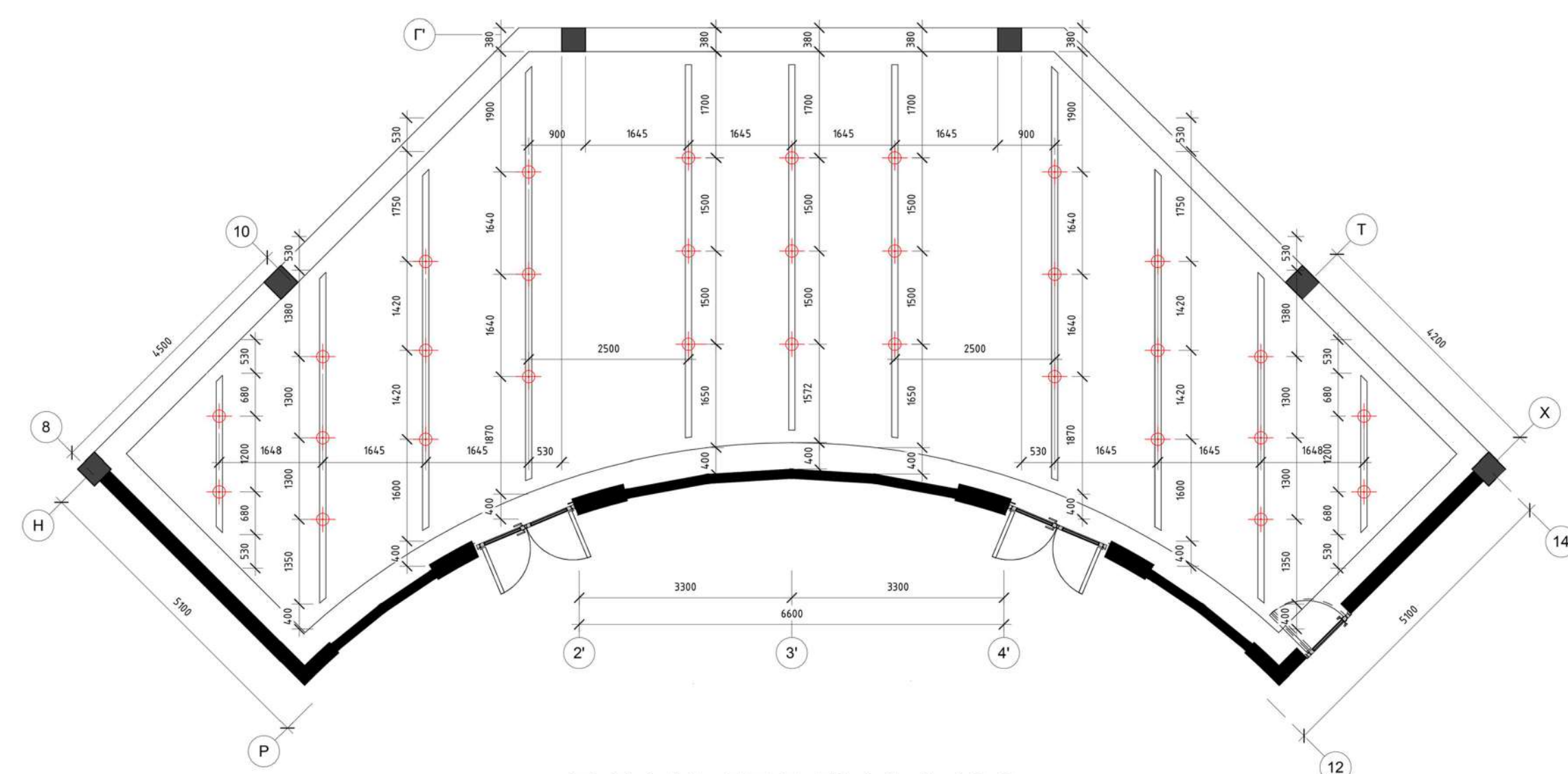
ПЛАН СТЕЛІ М 1:100
