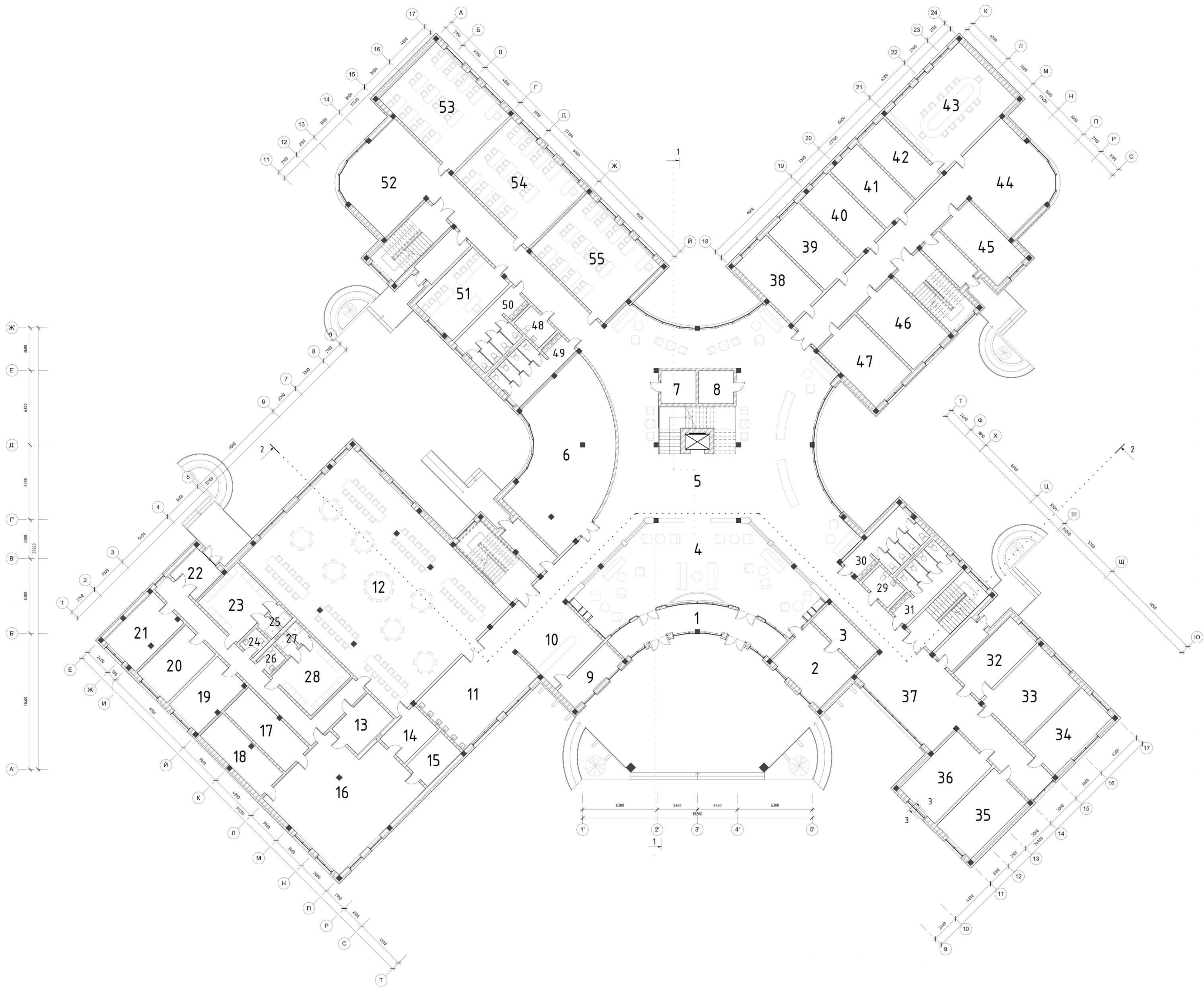
ПЛАН НА ВІДМІТЦІ +0.000 М 1:200
