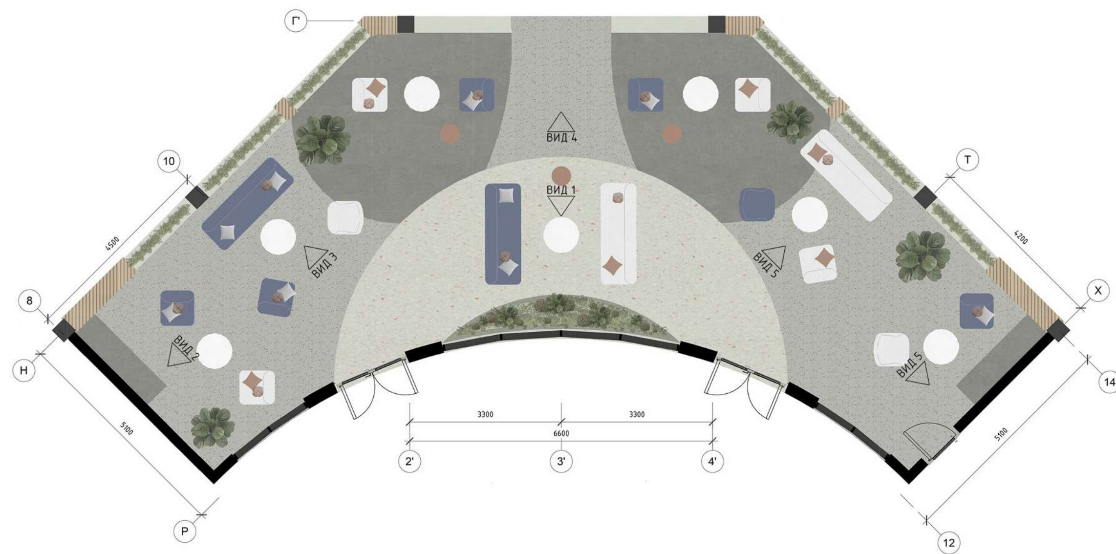
ПЛАН ПІДЛОГИ М 1:100
