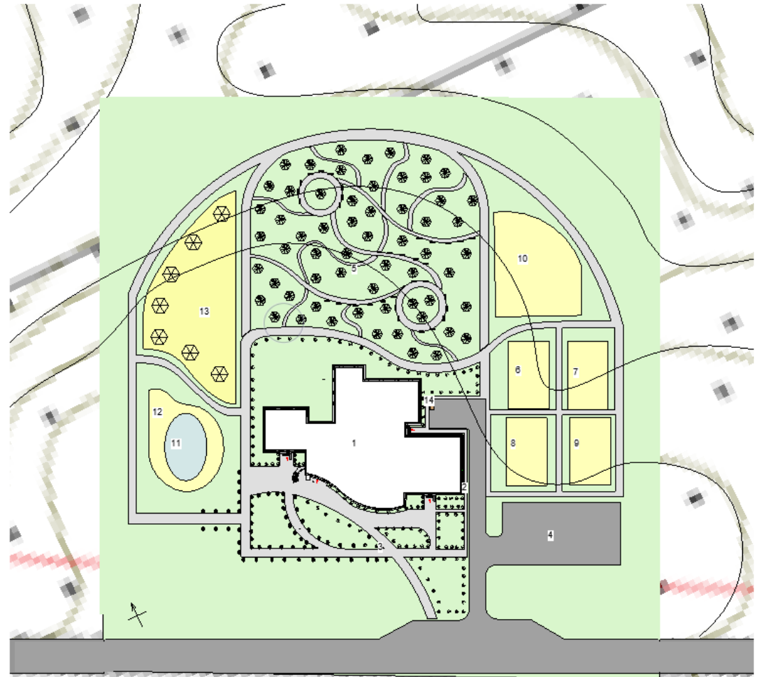
7 Ген. план 1:500
