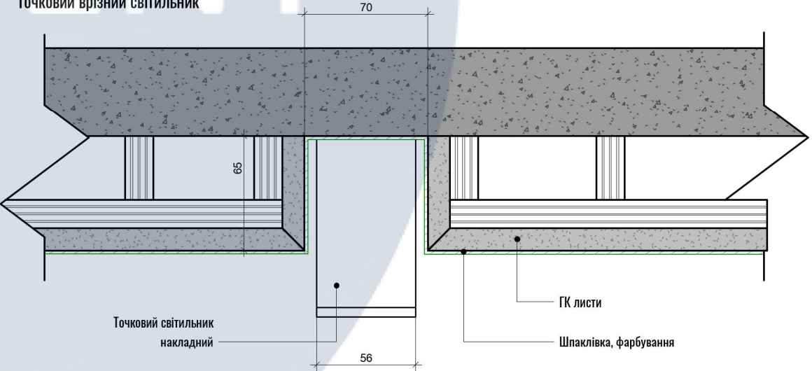
Точковий врізний світильник
