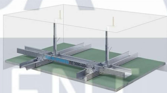
Підвісна гіпсокартонна стеля
