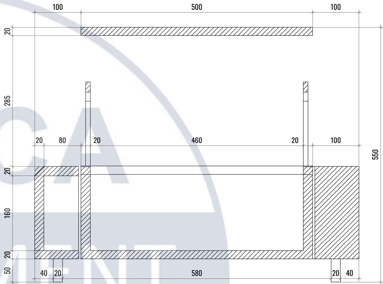
Вузол М 1:5
