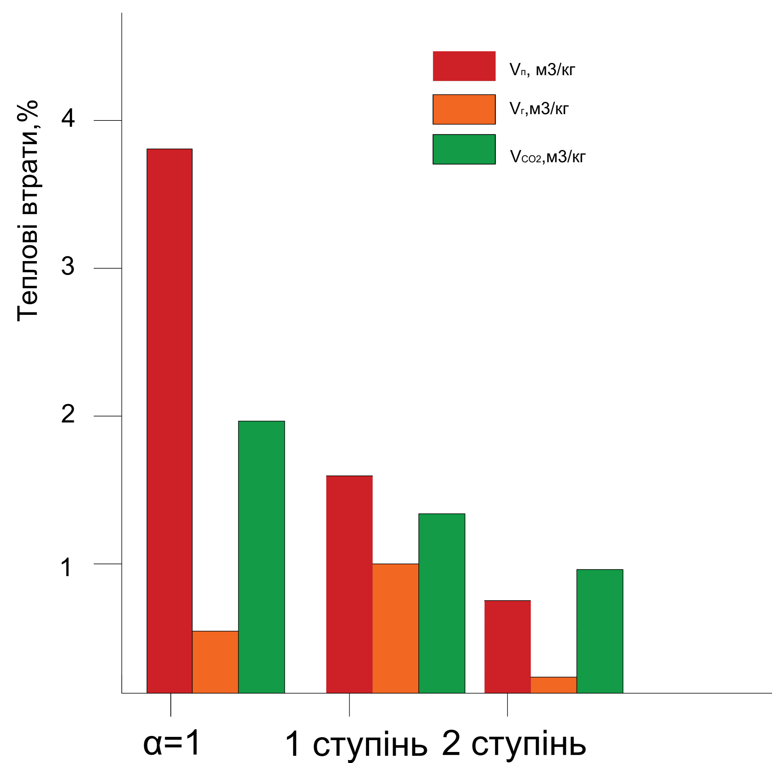
Теплові втрати
