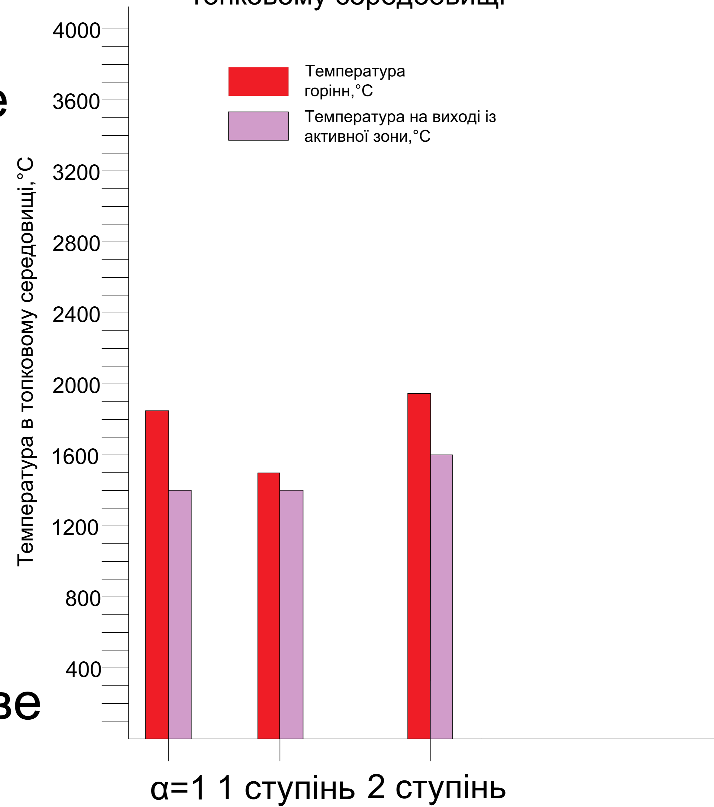
Температура горіння в топковому середовищі
