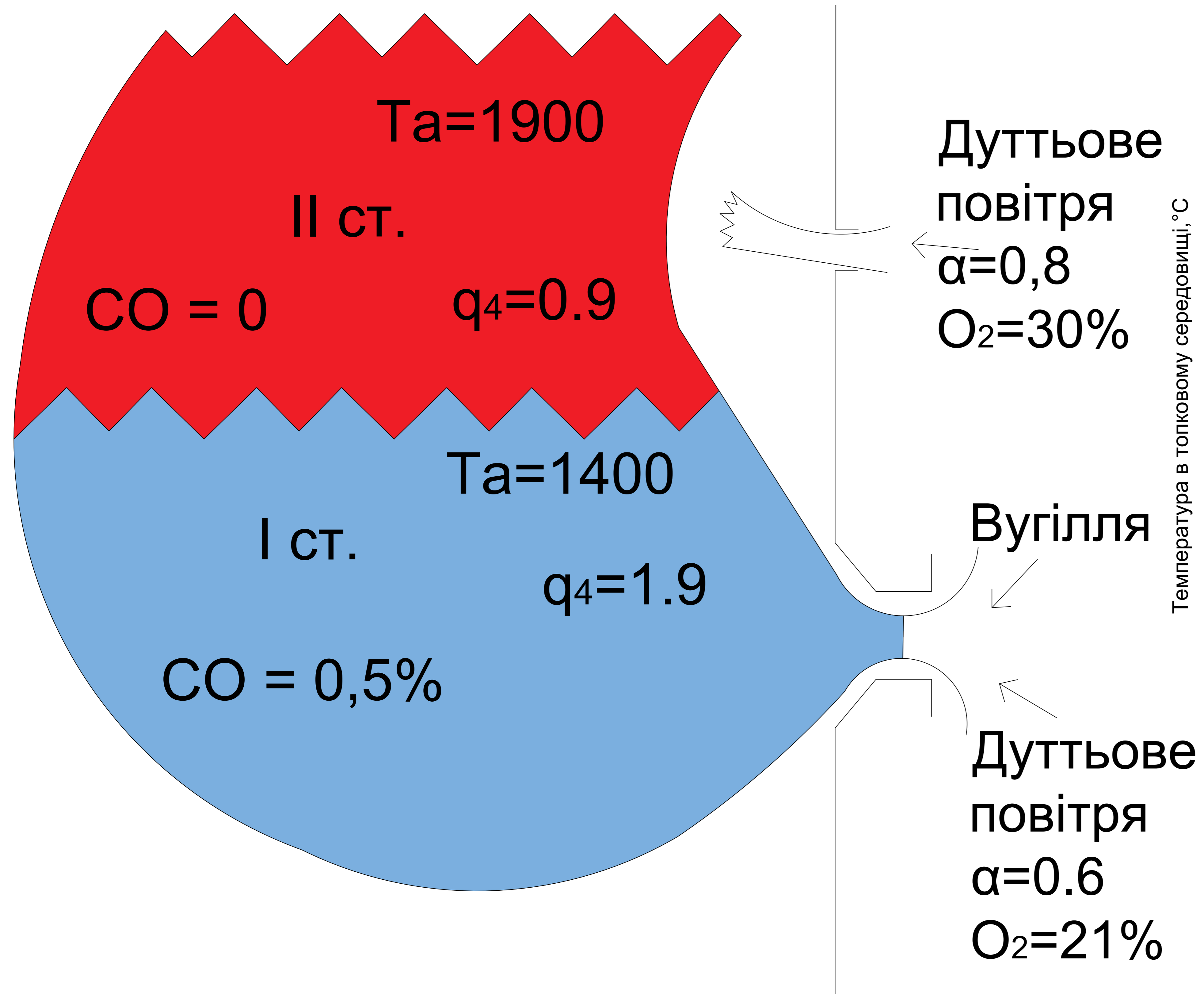
Теплові втрати
