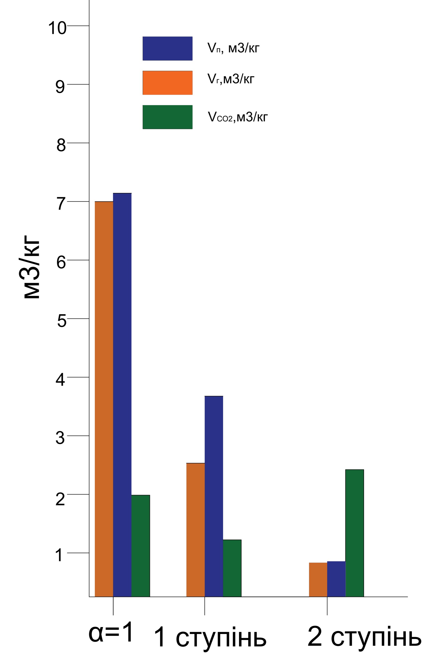
Об'єм димових газів та дуттьового повітря
